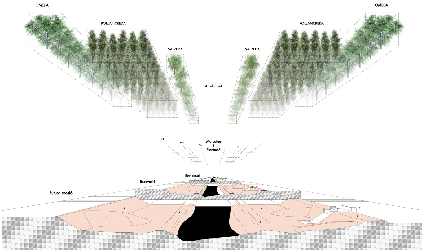
1. Espigó: Excavació + Hidrosembra 2. Dic: Capes superposades de terra compactada de 10 cm 3. Tolló: Excavació + Hidrosembra 4. Plano d'inundació: Excavació + Marcatge + Plantació Pollanques a arrel nua 5. Comporta (detall adjunt)
