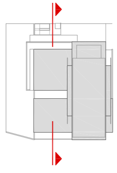
SECCIÓ 1 E: 1/150
