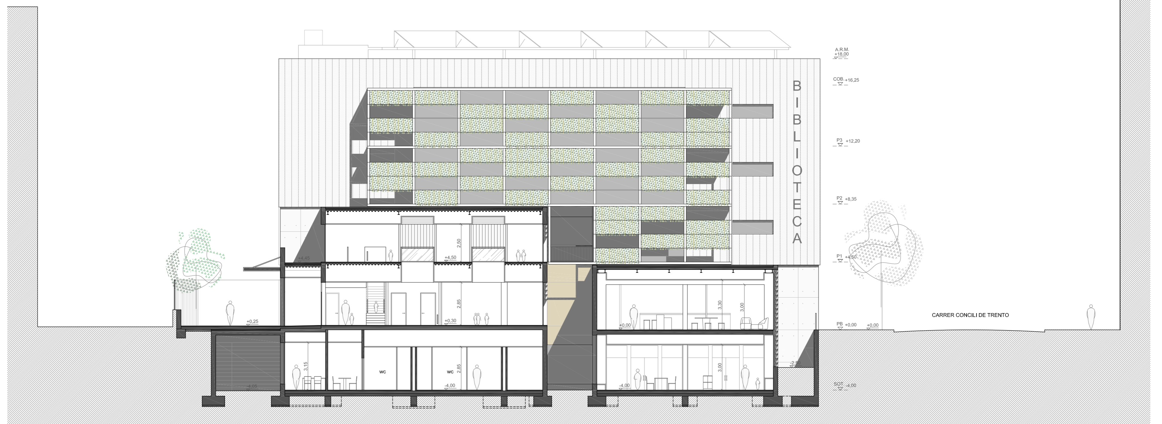
ALÇAT INTERIOR E: 1/150
