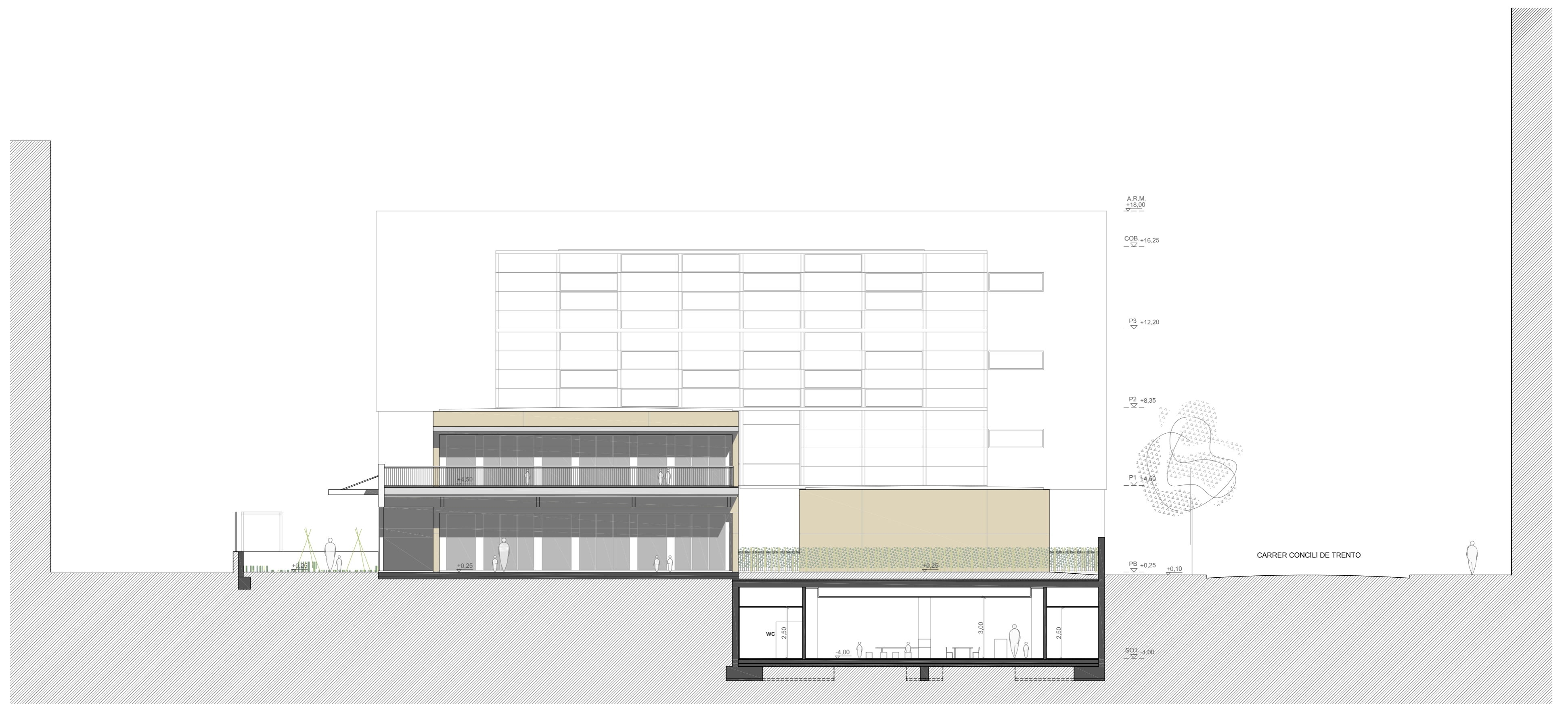
ALÇAT PATI ESCOLA E: 1/150
