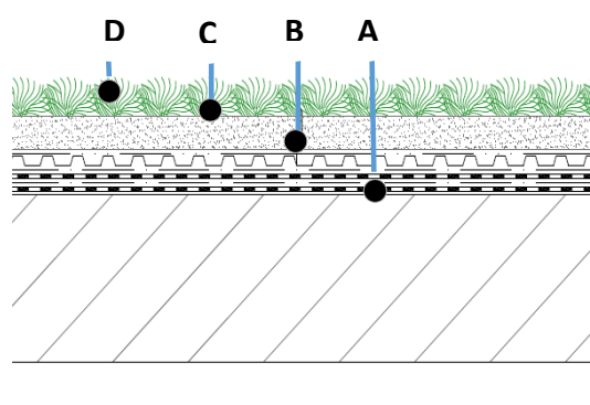
Fig. 5 Distribució de les sondes de recollida de dades higròtermiques en una solució tipus de coberta enjardinada
