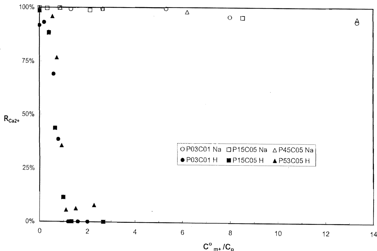
Figura 4. Influència de l'addició de sodi i àcid en el rebuig de calci. C_{m+}^0 concentració de Na^+ o H^+ addicionats. C_p concentració de polímer. Símbols blancs: addició de sodi, símbols negres: addició d'àcid.
