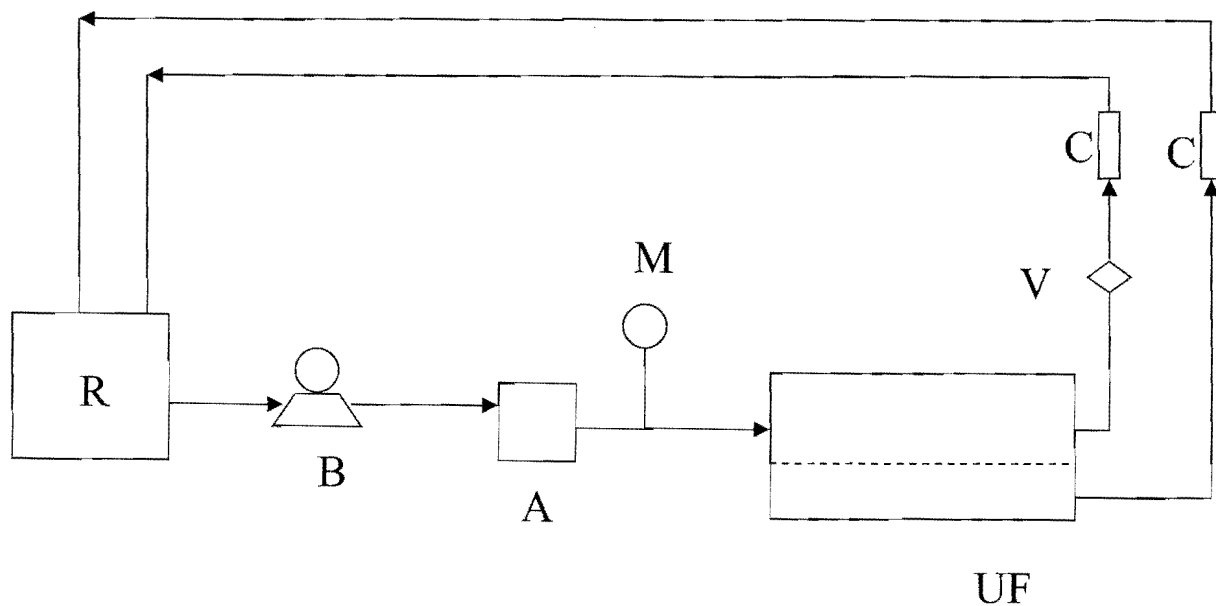
Figura 3. Dispositiu experimental. A: amortidor d'oscil·lacions de pressió. B: bomba impulsora. C: cabalímetre. M: manòmetre. R: tanc de reserva. V: vàlvula reguladora. UF: cèl·lula d'ultrafiltració.
