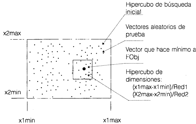
Figura 4. Búsqueda aleatoria.
