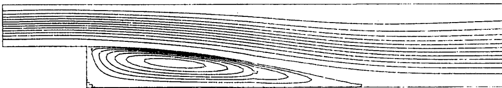
Figura 3. Visualización de algunas líneas de corriente (cálculos realizados utilizando la Biblioteca MODULEF). Valor del número de Reynolds: 190.
