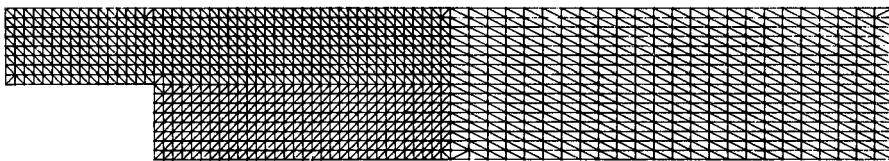
Figura 2. La triangulación utilizada (técnica MODULEF; elemento finito de Thomasset, P_1 —no conforme, base con divergencia nula).
