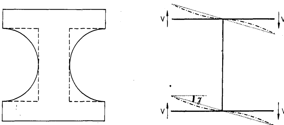
Figura 4. Esquema para el cálculo de la rigidez transversal frente al esfuerzo cortante, por la analogía de la viga Vierendeel.
