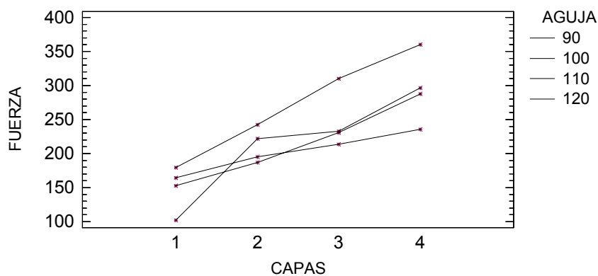
FIGURA 14: Interacción capas-aguja en el tejido de 400 g/m 2 .
