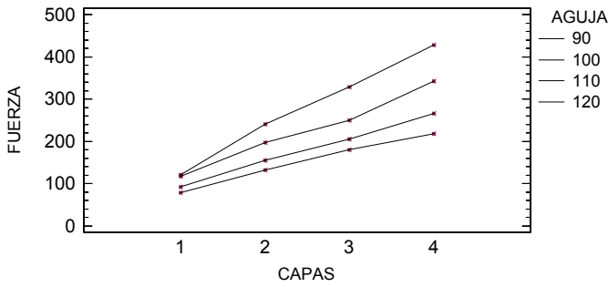
FIGURA 11: Interacción capa-aguja en tejidos de 305g/m 2 .
