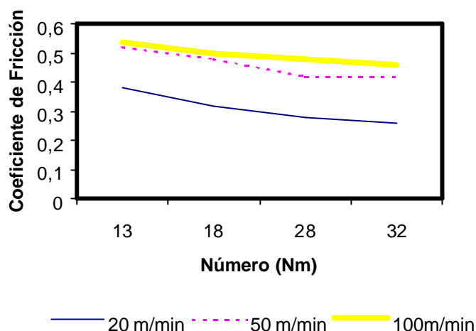
FIGURA 2: Efecto del número en el coeficiente de fricción de hilos 100% acrílicos. Material: cerámica. Ángulo de rozamiento: 90°.
