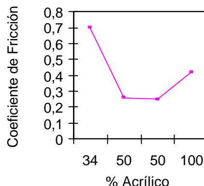
FIGURA 3: Efecto de la composición (Acri/Mo) en el coeficiente de fricción de un hilo. Material: Acero. Velocidad: 20 m/min. Ángulo de rozamiento: 90°.
