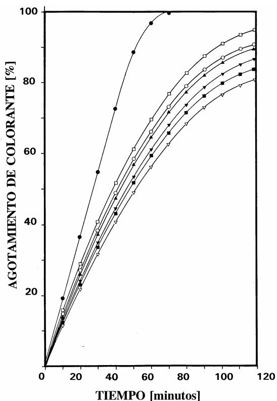
FIGURA 4A: Cinéticas de agotamiento del colorante Acid Yellow 129 sobre lana no tratada a diferentes concentraciones de PC, la concentración de colorante permaneciendo constante (1.0 % sobre peso de fibra). Concentración de PC (% sobre peso de fibra), 0 (●), 0.56 (∇), 1.70 (▼), 2.83 (◊), 3.97 (□), 5.10 (▲), 6.81 (■).
