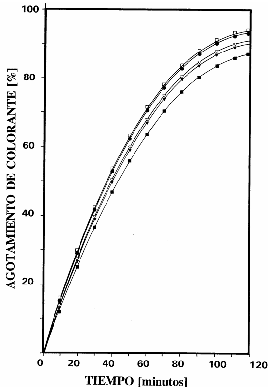
FIGURA 4B: Cinéticas de agotamiento del colorante Acid Yellow 129 sobre lana tratada a diferentes concentraciones de colorante, la concentración de PC permaneciendo constante (2.27 % sobre peso de fibra). Concentración de colorante (% sobre peso de fibra), 0.10 (■), 0.30 (∇), 0.50 (□), 0.60 (●), 0.90 (▼).
