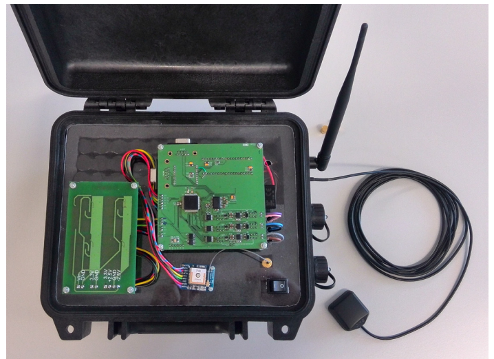
Fig. 1 Equipo de adquisición sísmica volcánica
