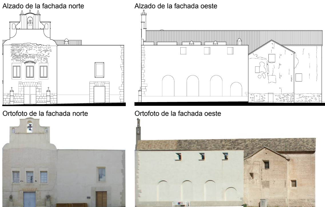
Figura 7. Alzados y ortofotos de las fachadas norte y oeste
