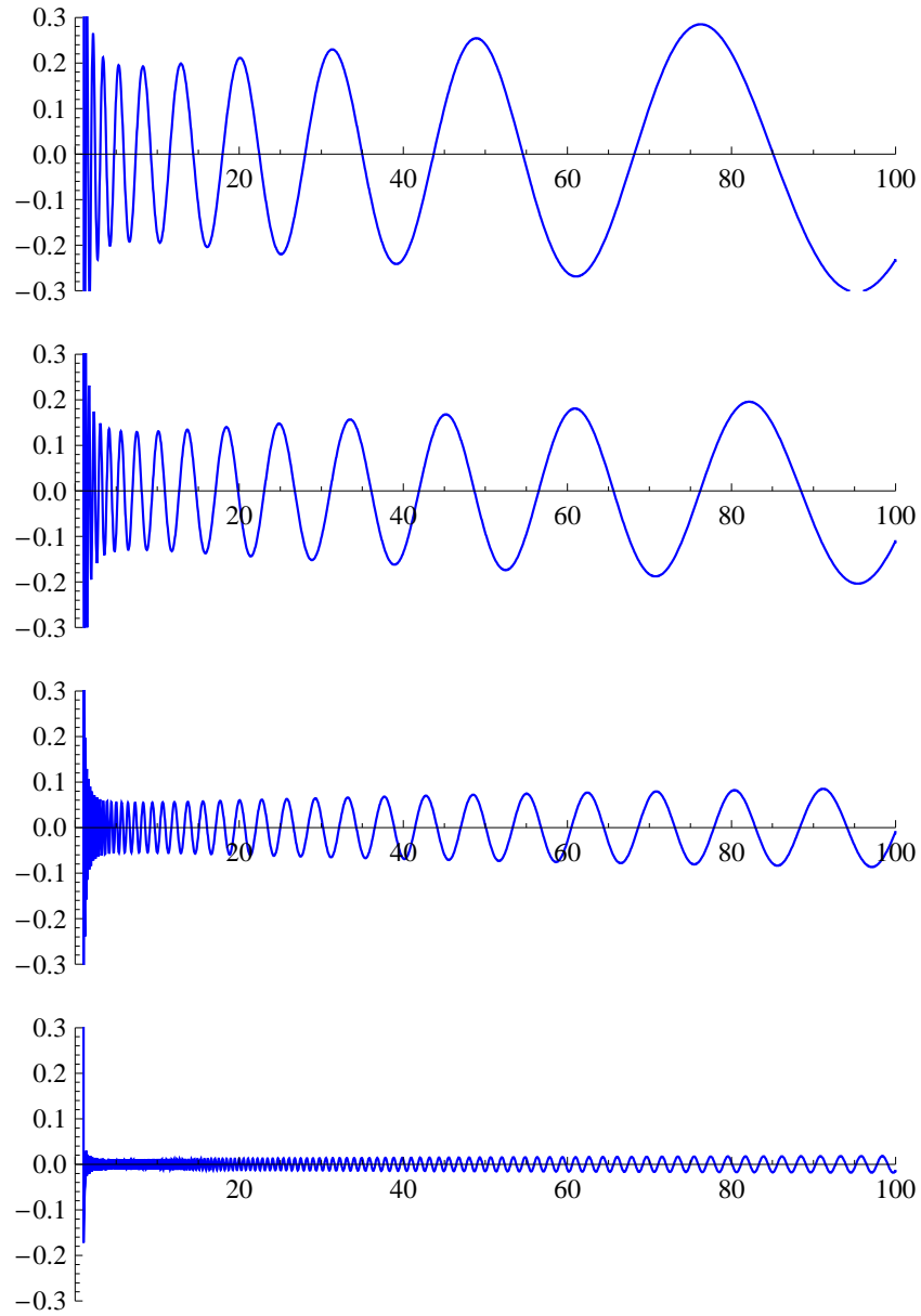
FIGURA 4. Termes oscil·latòris -\text{Li}(x^\rho) - \text{Li}(x^{1-\rho}) corresponents als parells d'arrels nùmeros 1,2,10 i 100.
