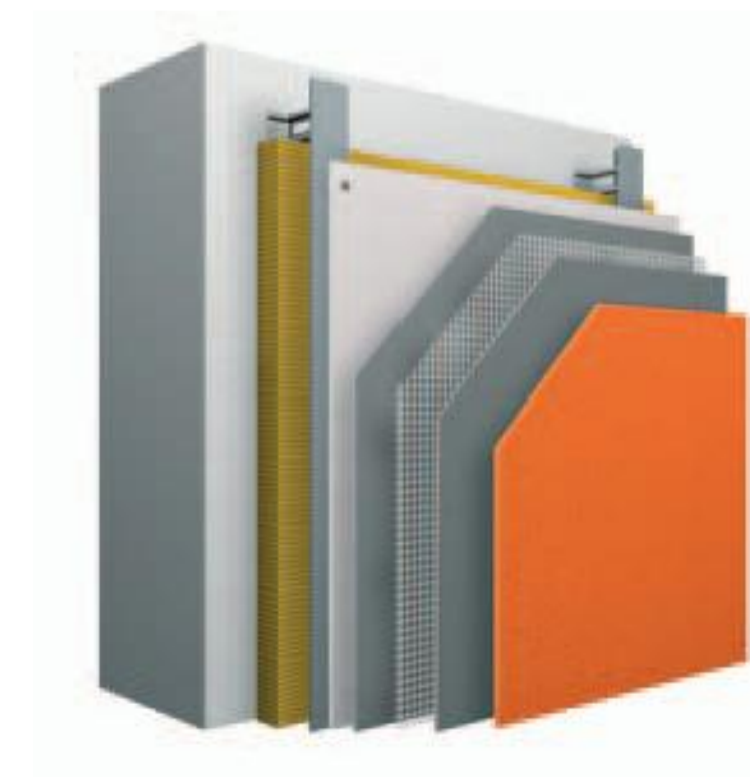
SISTEMA FAÇANA VENTILADA STO VENTEC
