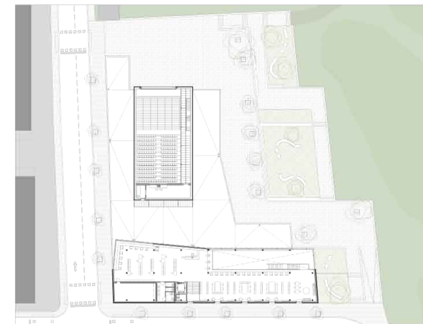
PLANTA PRIMERA
