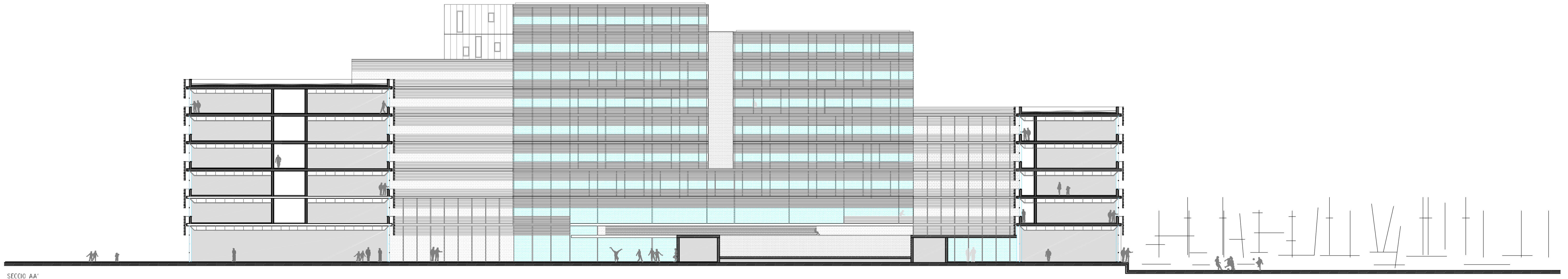
SECCIO AA'
