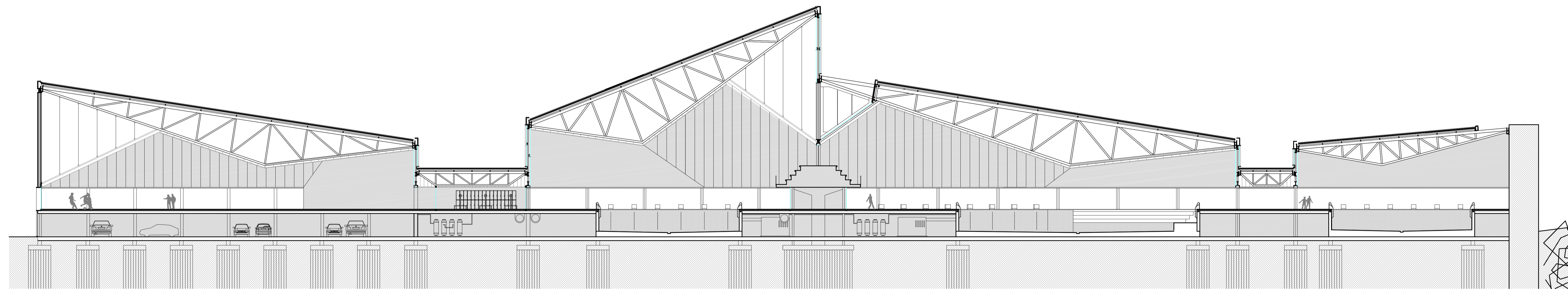
SECCIÓ BB'
