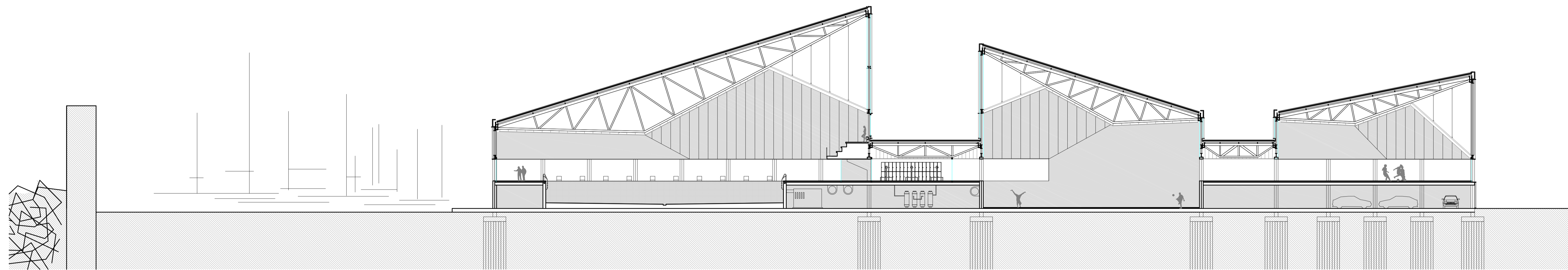
SECCIÓ AA'
