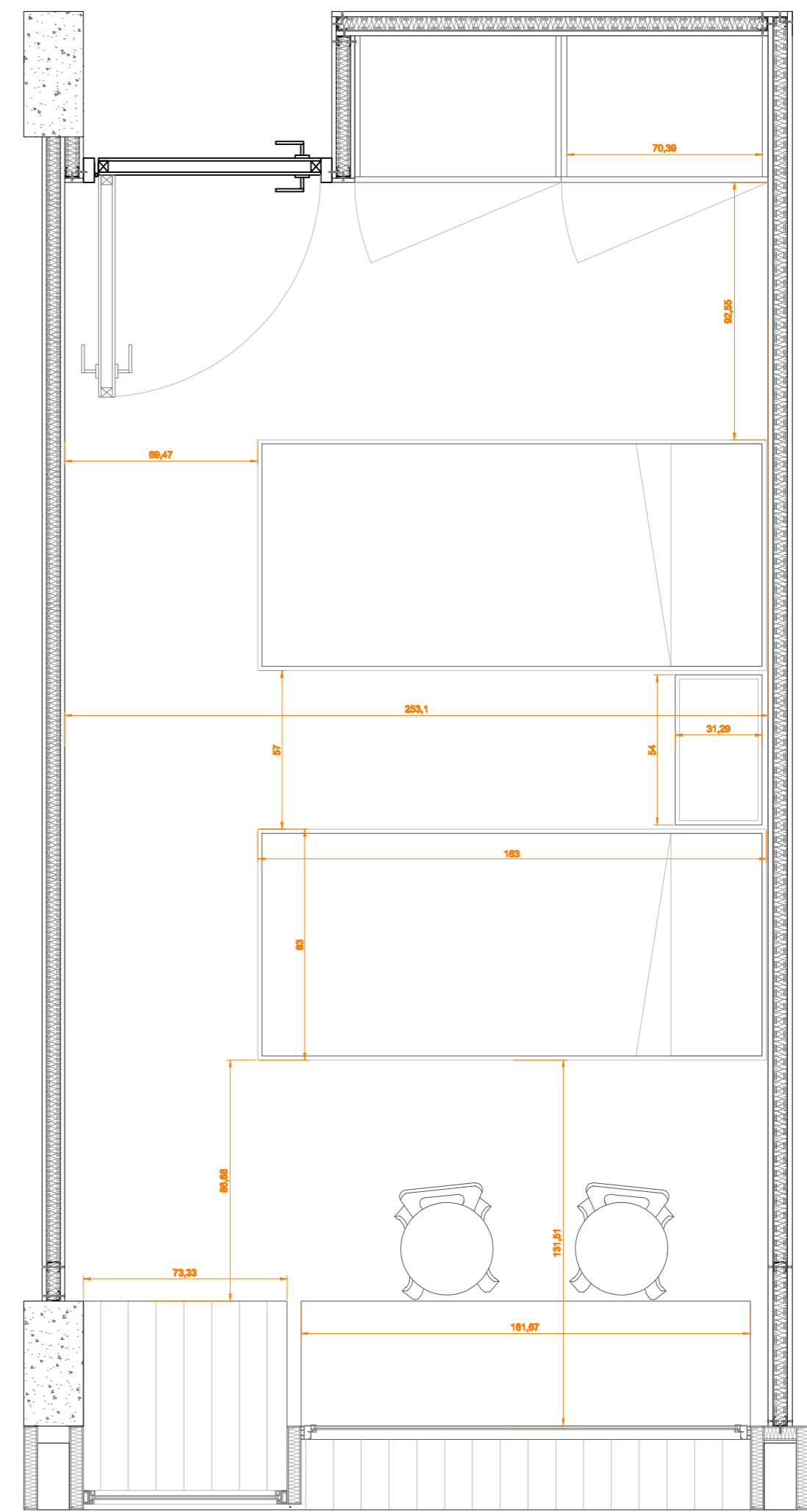
PLANTA E:1/20
