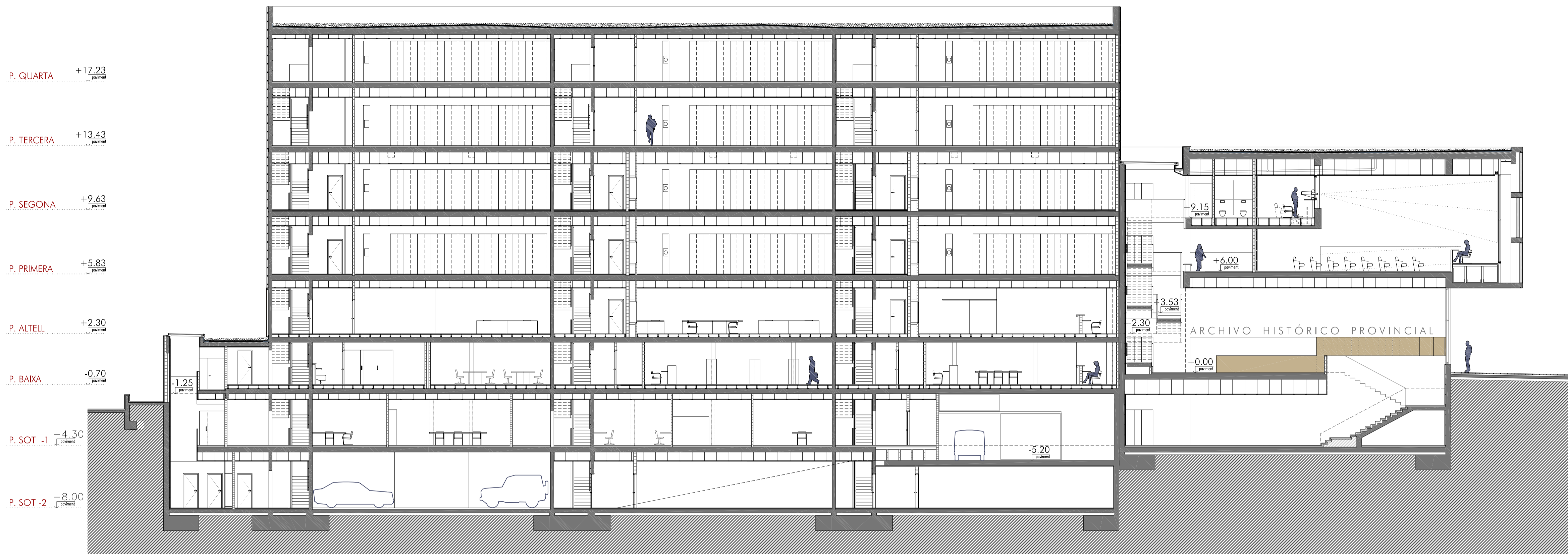
SECCIÓ L1
