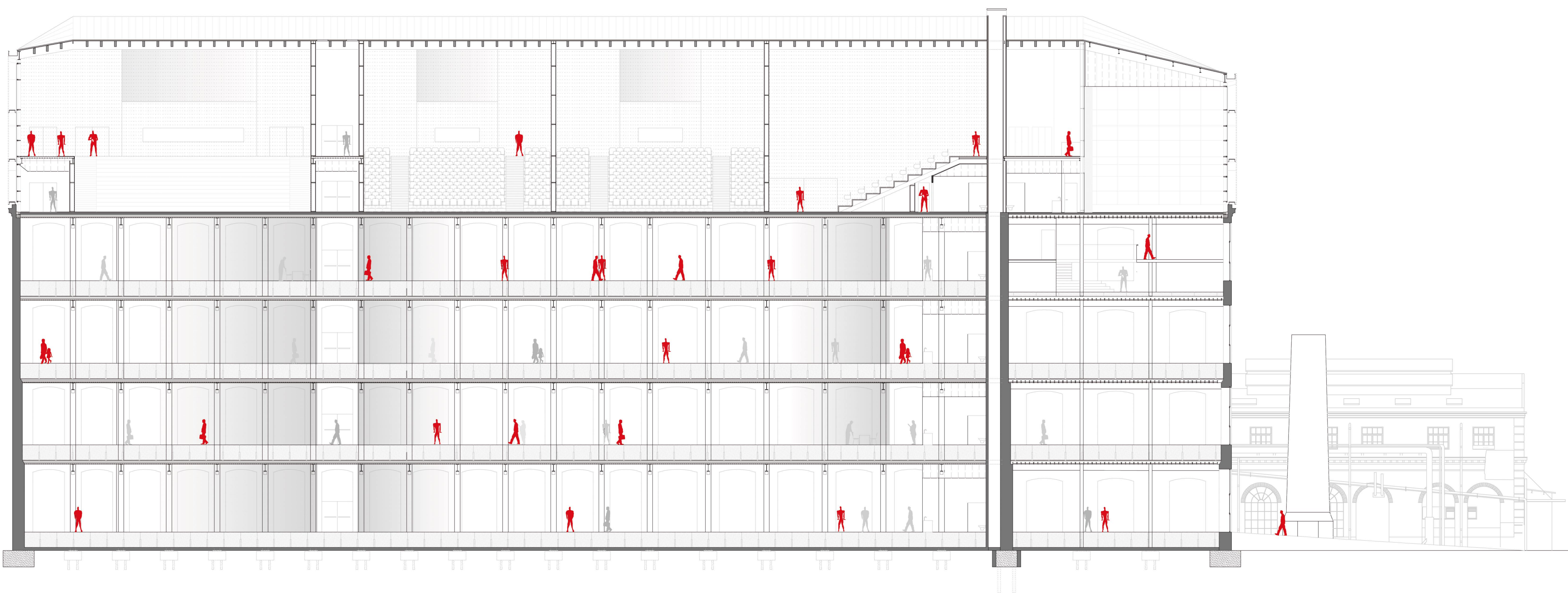
seccion e 1:200
