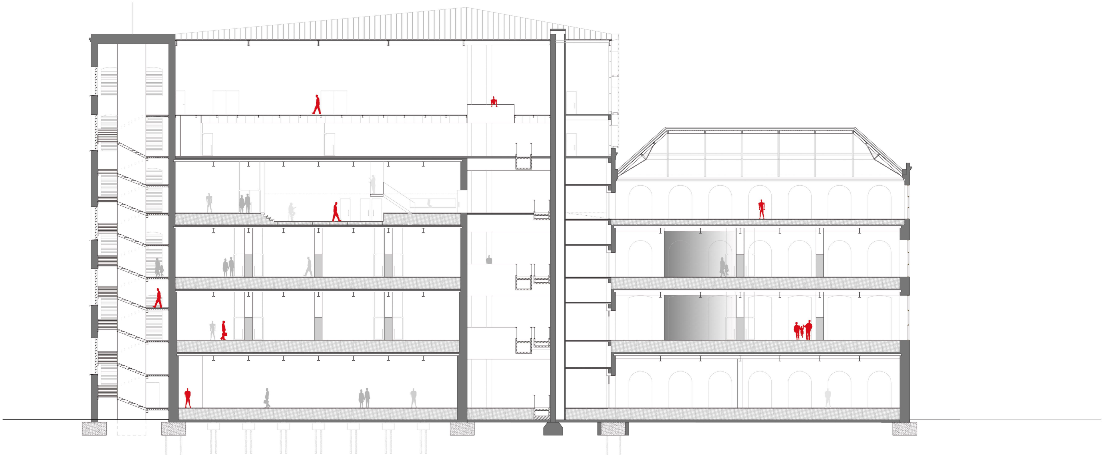
sección transversal 1:200
