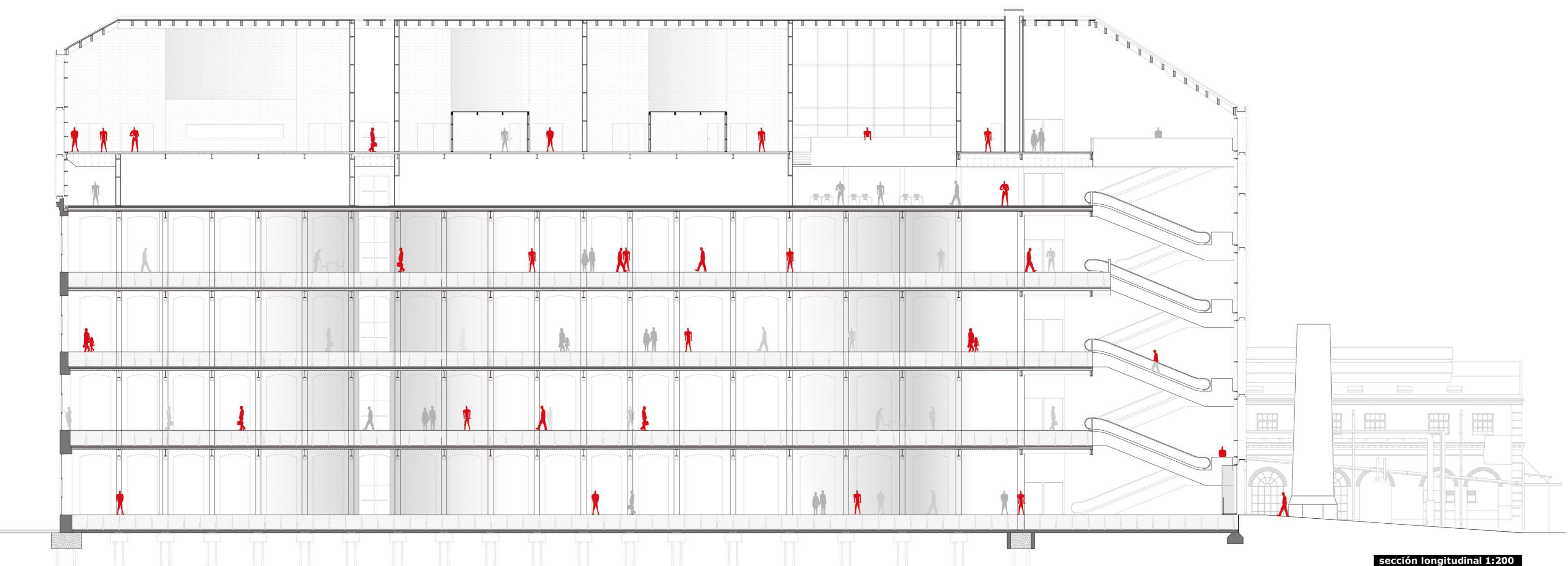
sección longitudinal 1:200
