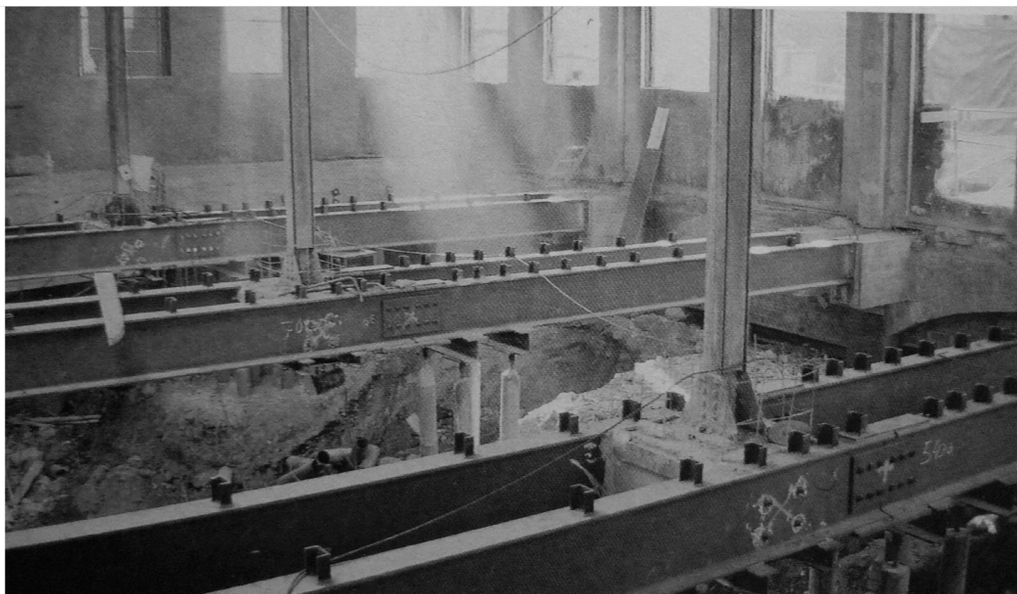
obras de ejecución de micropilotes
