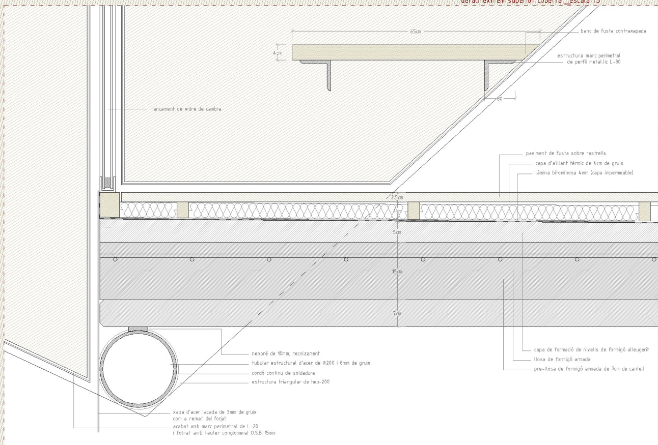
detall recolzament del forjat _escala 1:5
