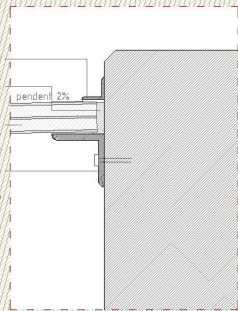
lluerni unió jàssera _escala 1:5
