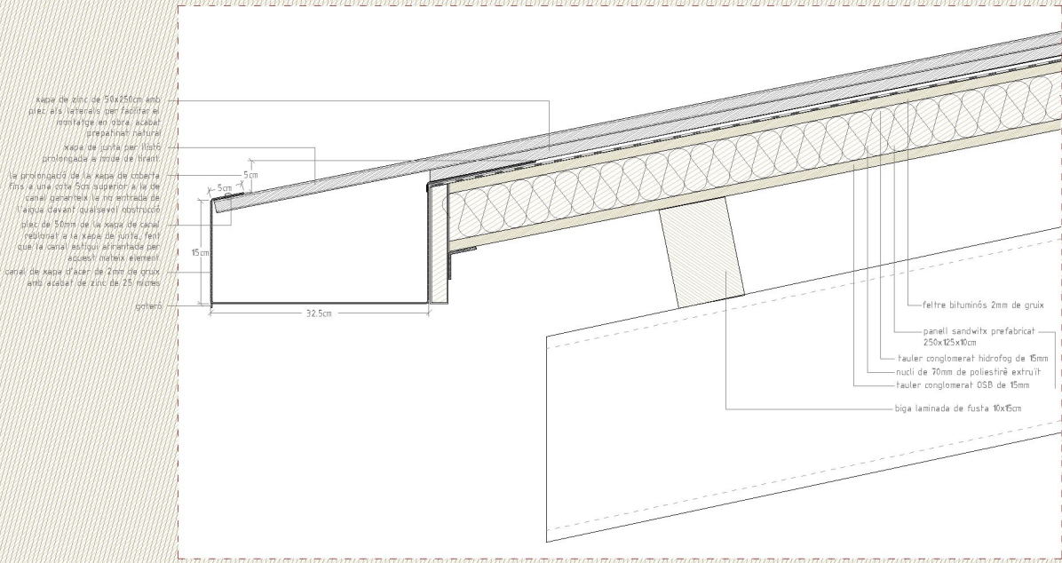
detall extrem inferior biga-canal _escala 1:5
