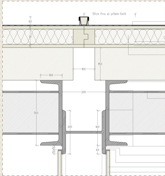
detall secció transversal biga _escala 1:5
