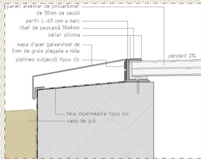
lluerni unió mur _escala 1:5
