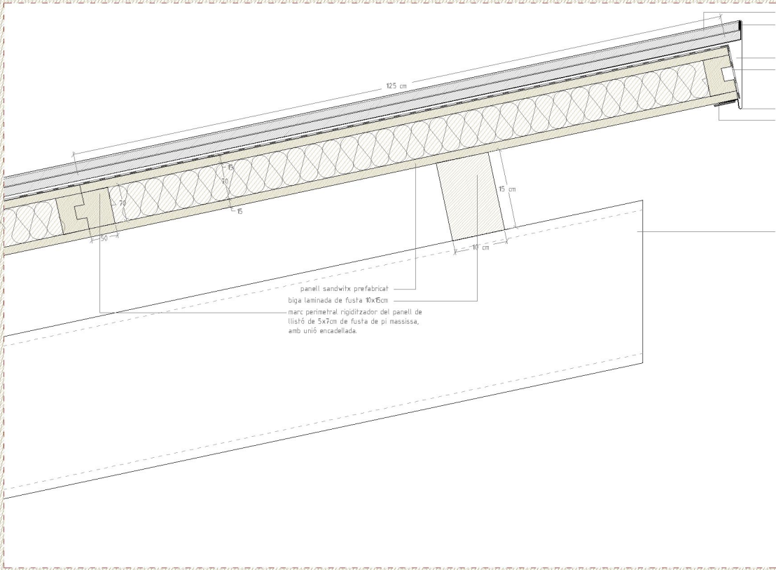
detall extrem superior coberta _escala 1:5
