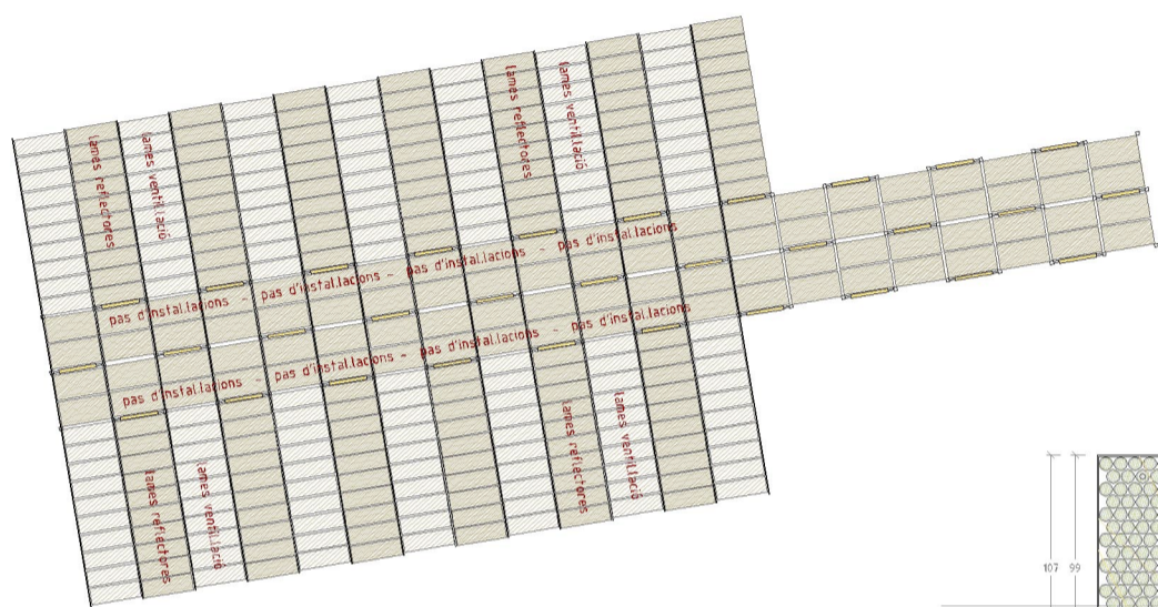
planta sostre cel ras estructural i de reflexió _escala 1:100
