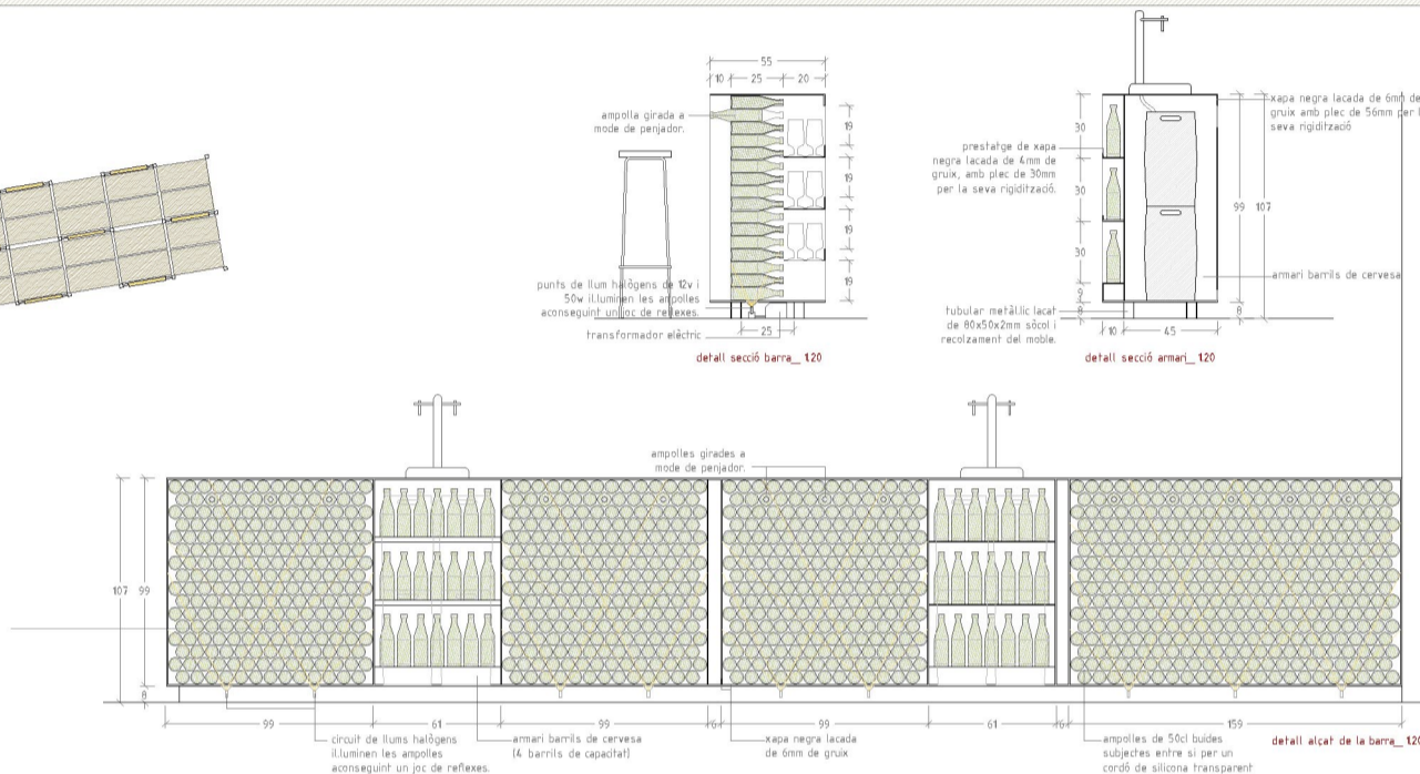
secció 3 cos principal_ celler barrils _escala 1:50
