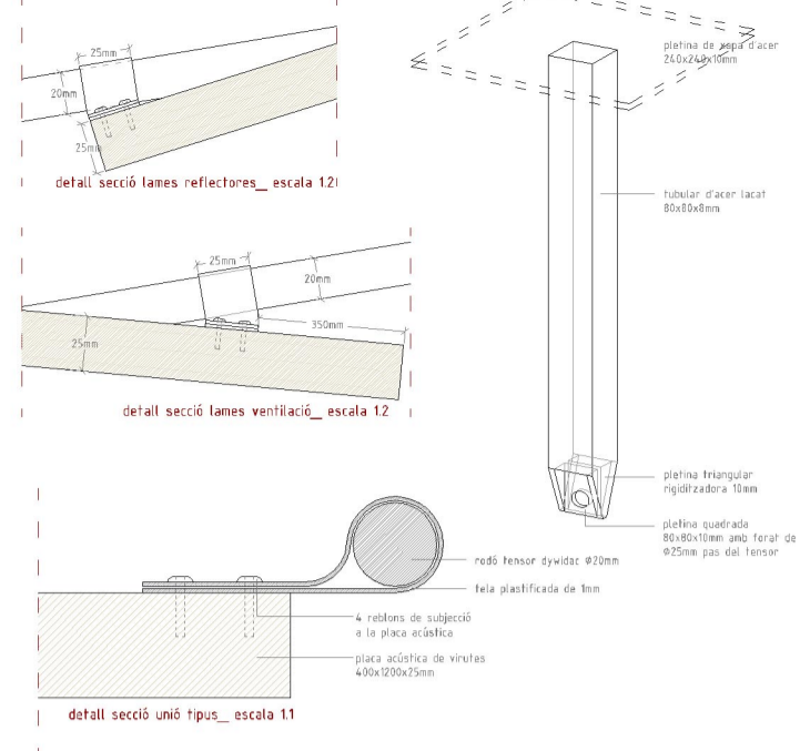
detalls definició cel ras estructural i de reflexió
