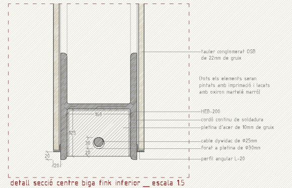
detall secció centre biga fink inferior _ escala 15
