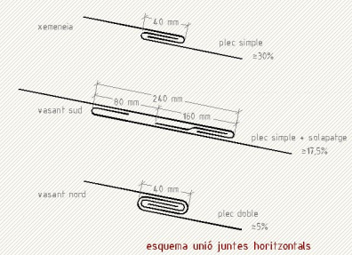
esquema unió juntes horitzontals
