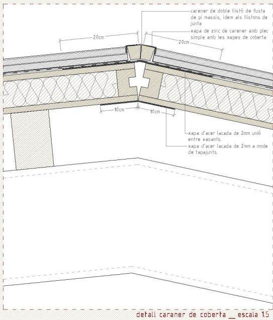
detall caraner de coberta _ escala 15
