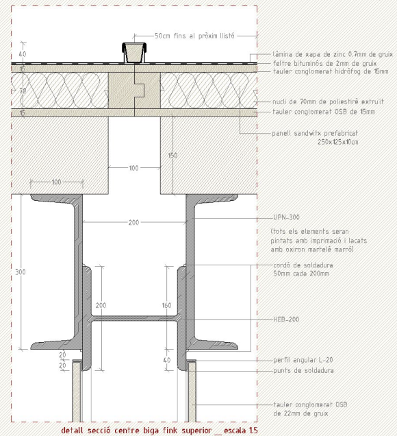
detall secció centre biga fink superior _ escala 15
