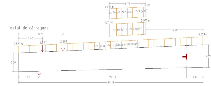
calcul estructural de la jàssera de façana 1:1000 1:200
