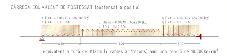
calcul estructural de la jàssera de façana 1:1000 1:200
