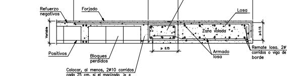
TRANSICIÓN A LOSA MACIZA DE IGUAL CANTO EN VOLADIZO
