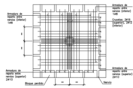
ARMADURA DE MONTAJE DE ÁBACO CENTRAL CON PILAR
