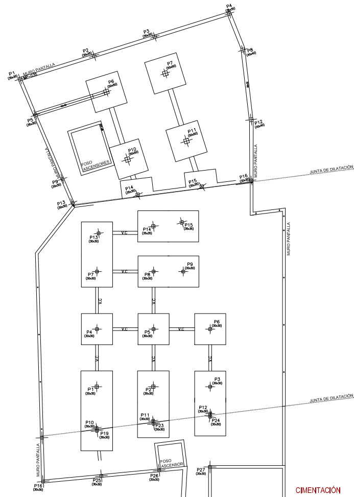
CIMENTACIÓN
