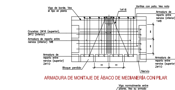
ARMADURA DE MONTAJE DE ÁBACO DE MEDIANERÍA CON PILAR
