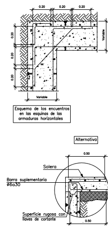
ENCUENTROS FOSO DE ASCENSOR
