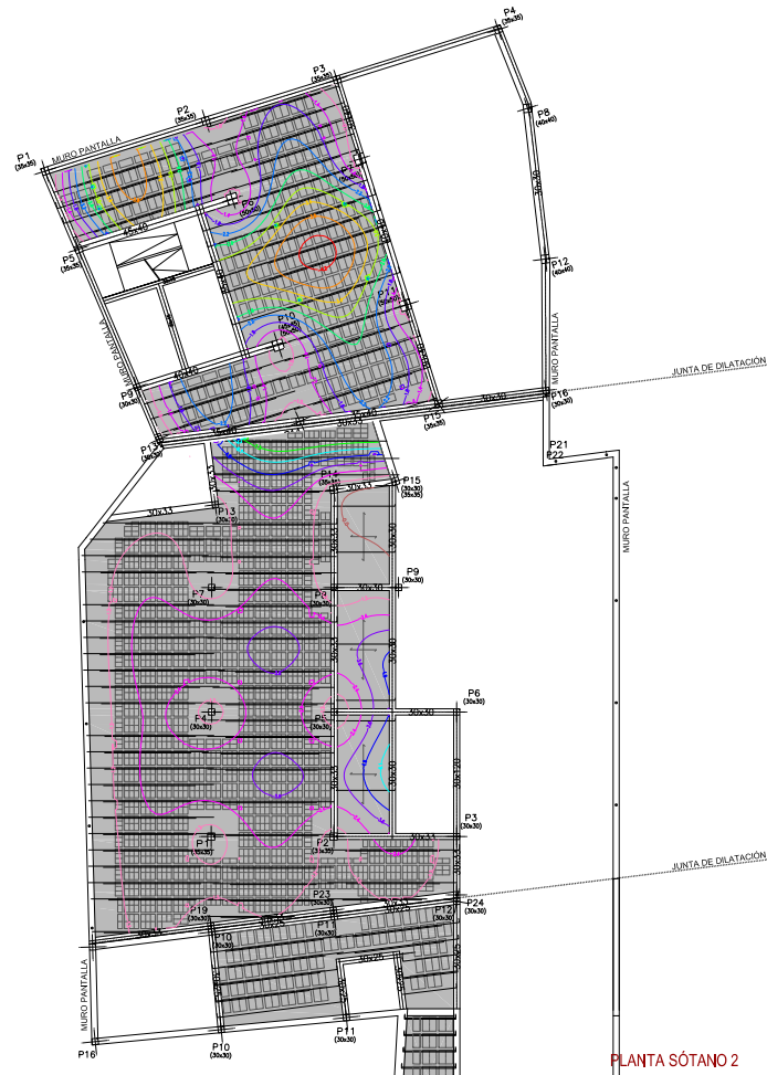
PLANTA SÓTANO 2
