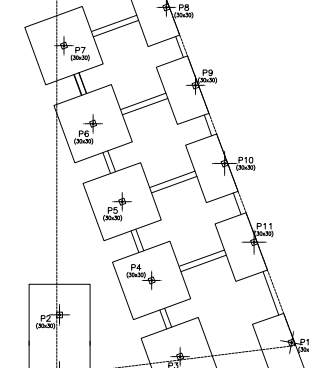
CIMENTACIÓN
