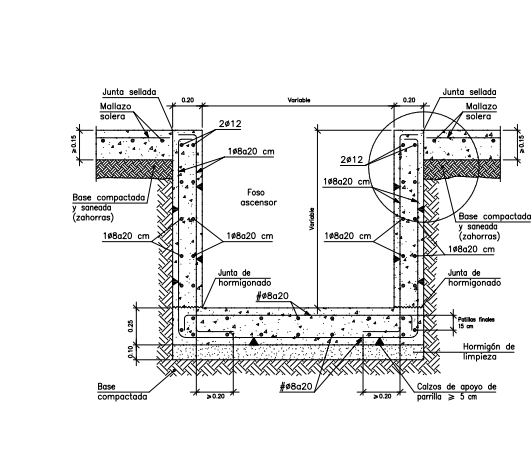
FOSO DE ASCENSOR
