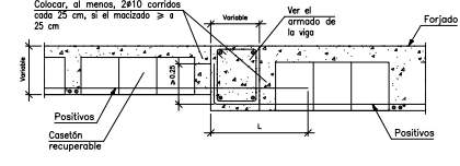
CAMBIO DE CANTO EN VANO INTERMEDIO
