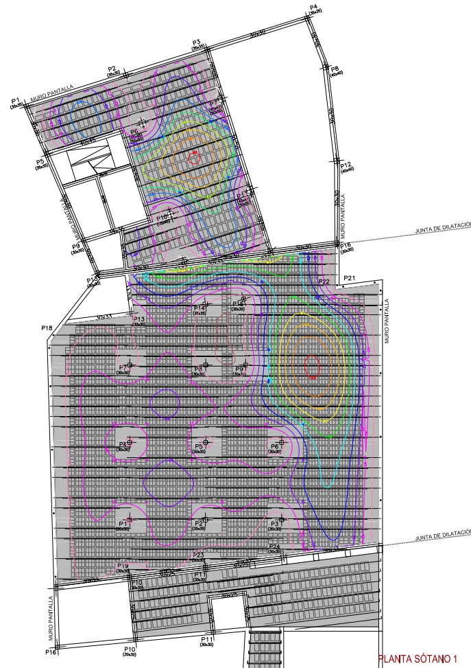
PLANTA SÓTANO 1
