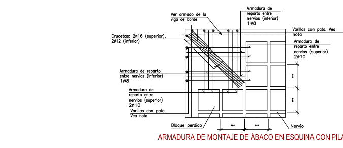
ARMADURA DE MONTAJE DE ÁBACO EN ESQUINA CON PILAR
