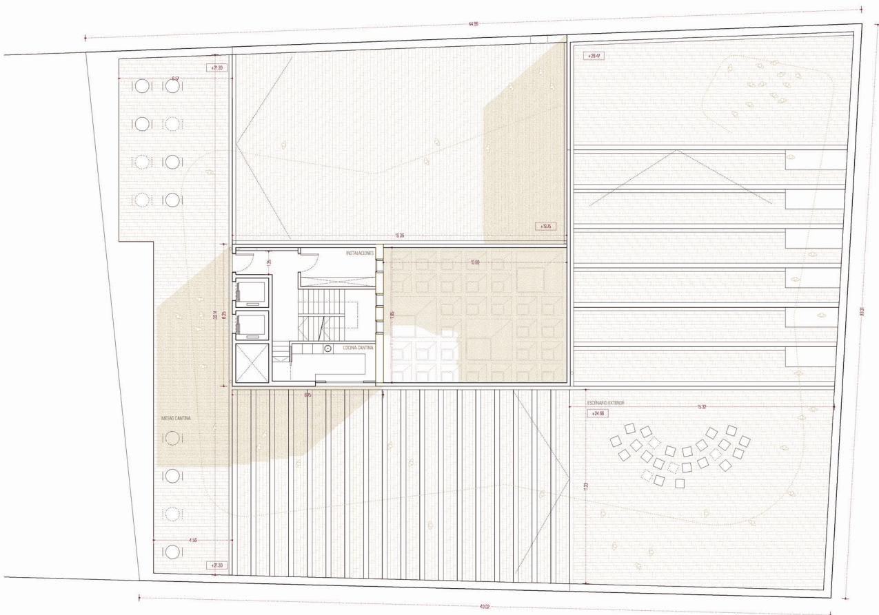
acceso cubierta (+21.30)
