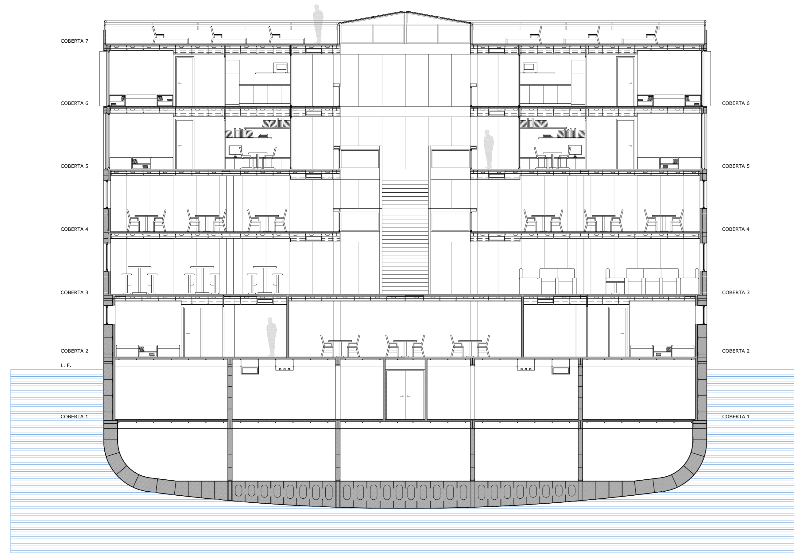
SECCIÓ TRANSVERSAL C - C'
