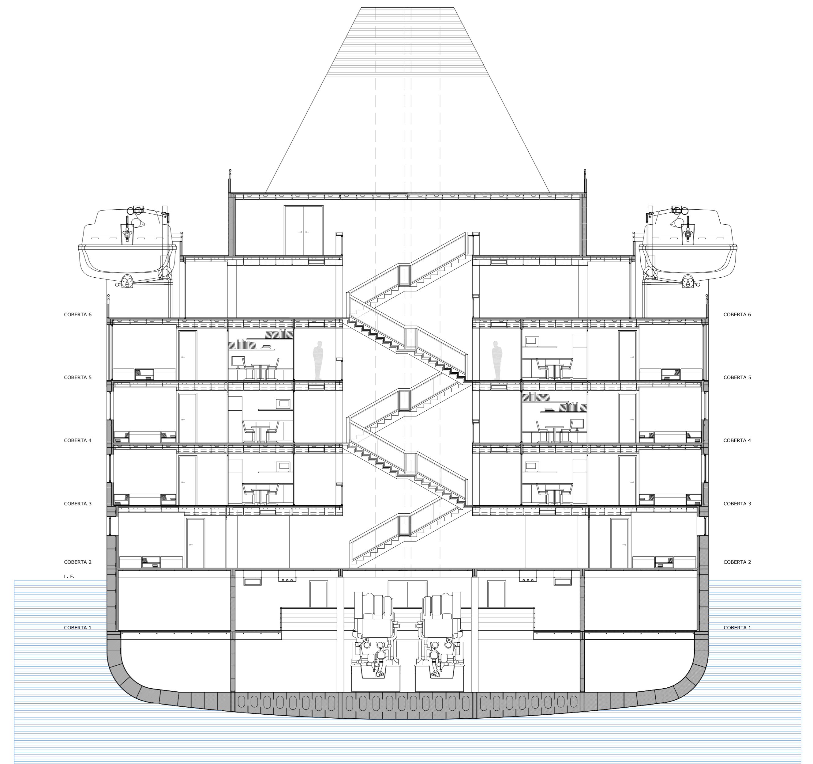
SECCIÓ TRANSVERSAL D - D'
