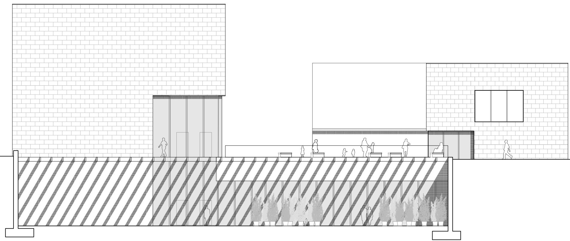
G-G' - ALZADO SUROESTE
