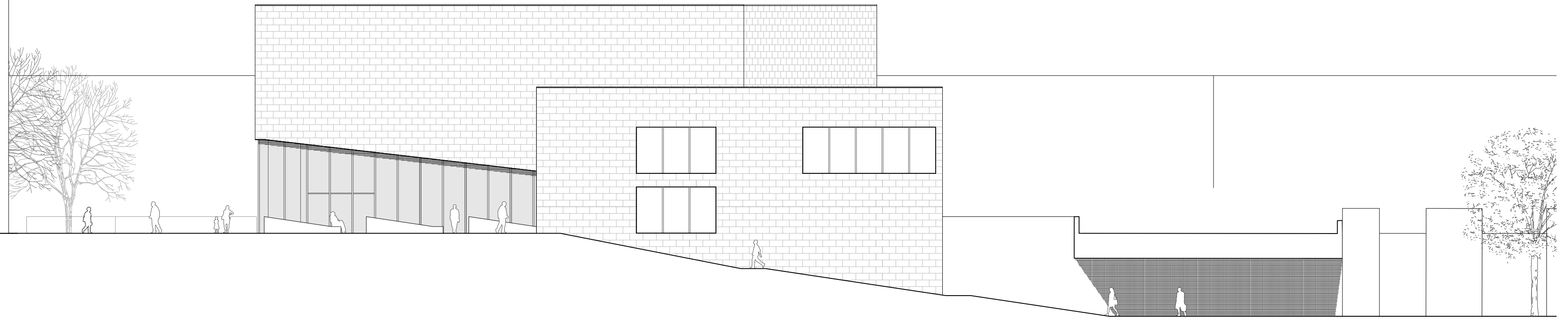
H-H' - ALZADO SURESTE
