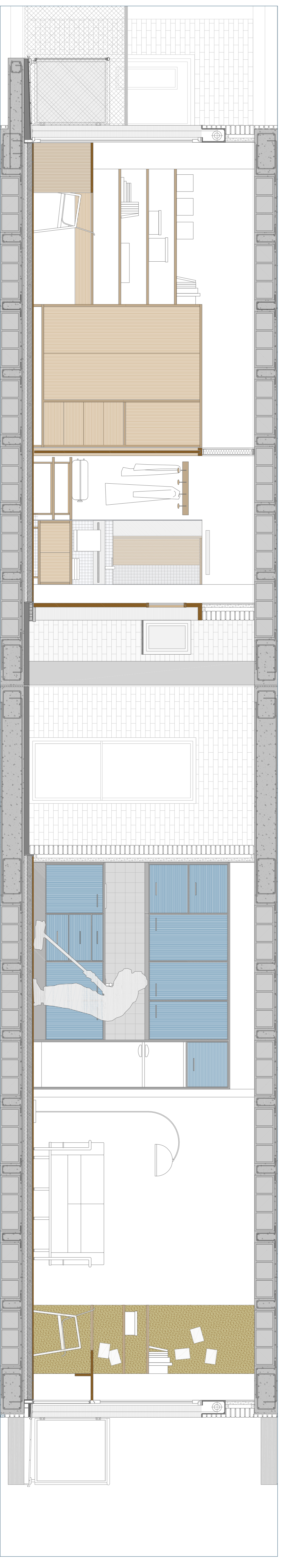
SECCIÓ a - a'
