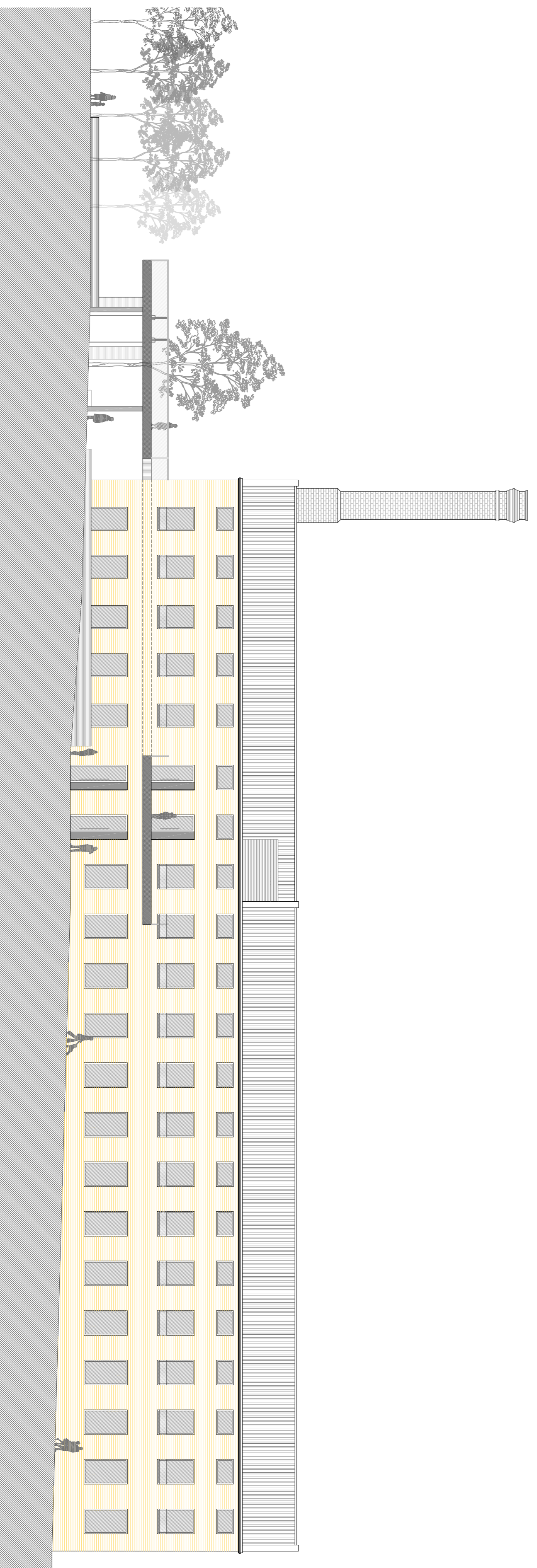
Alçat G-G'
