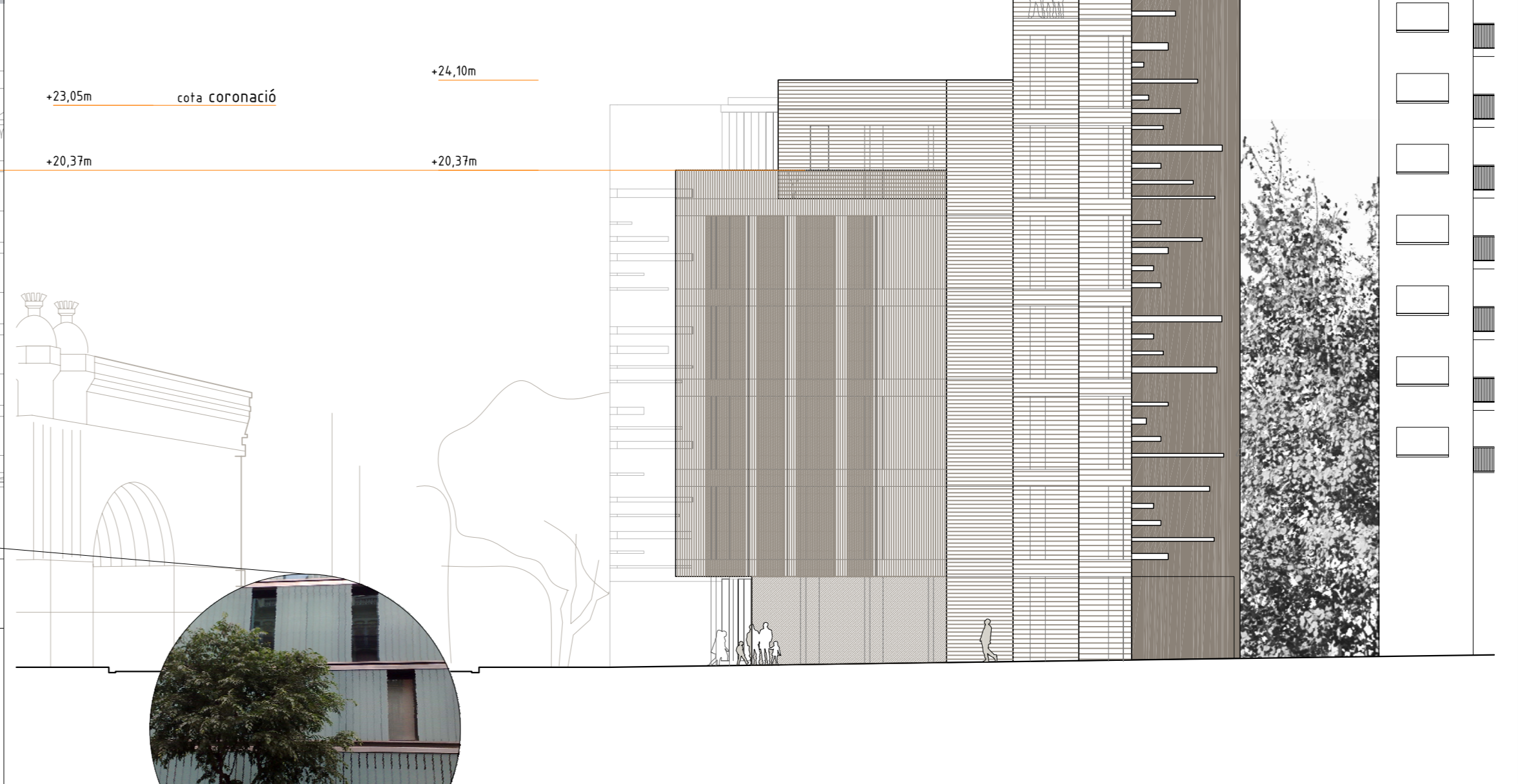
Alçat Hotel des de c/Ali-Beí
