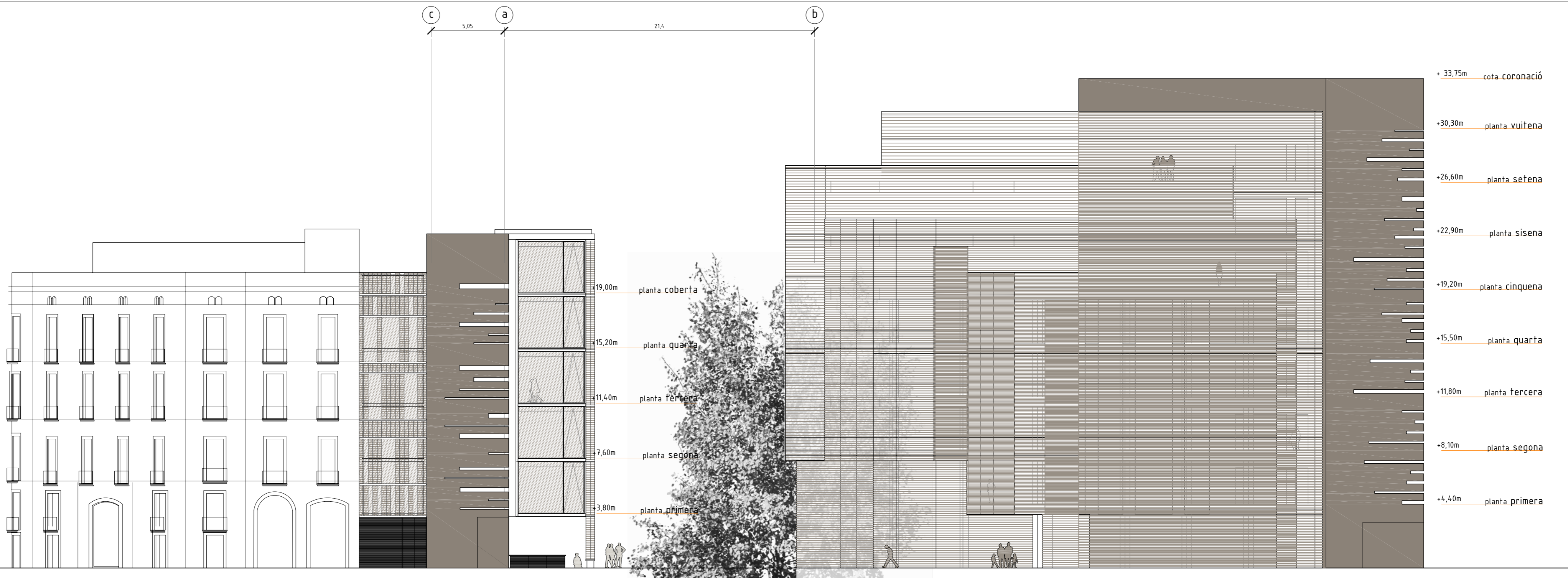
Alçat Avinguda de Vilanova
