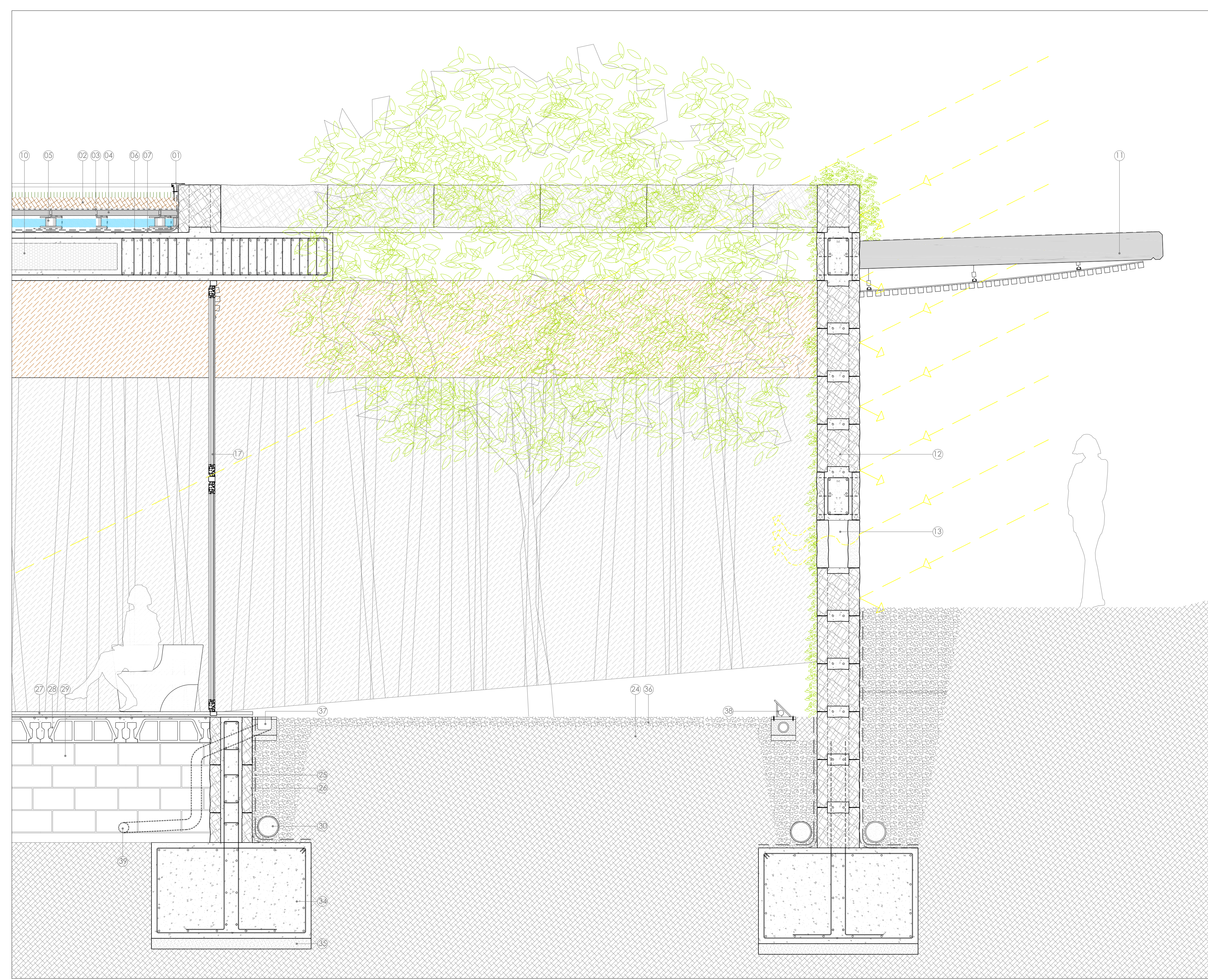
DETALL H
