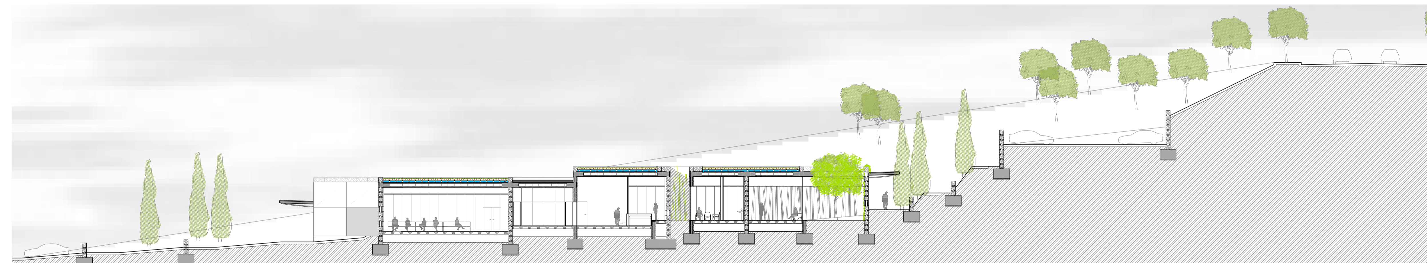
SECCIÓ LONGITUDINAL 3
