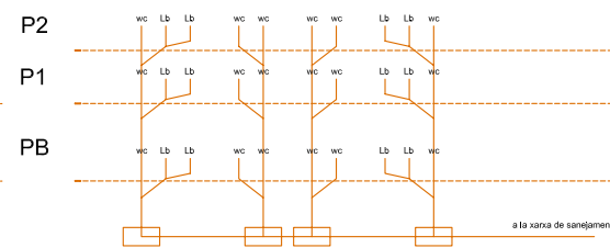
ESQUEMA DE SANEJAMENT DEL CENTRE CÍVIC
