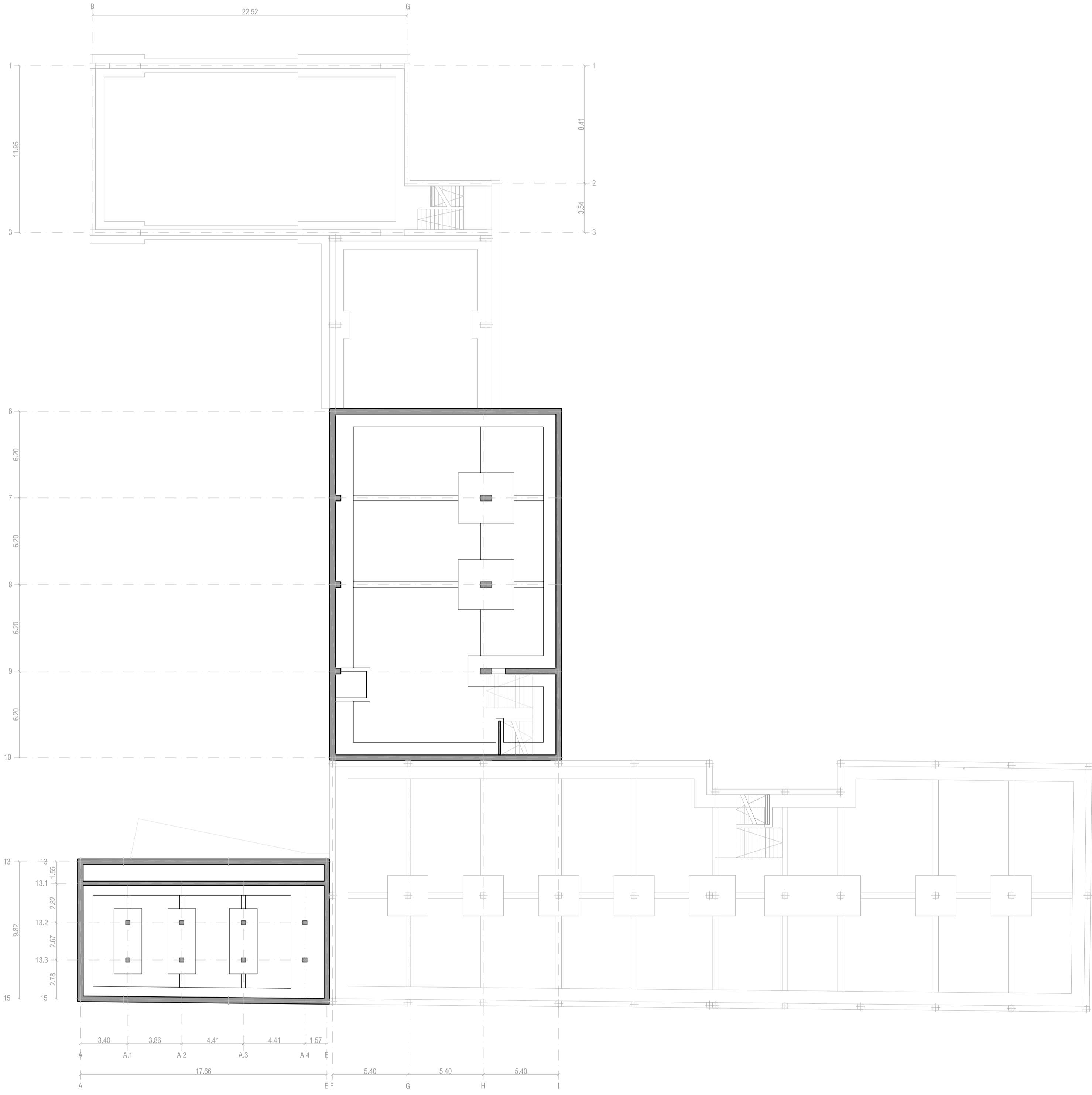
FONAMENTACIÓ P-1
