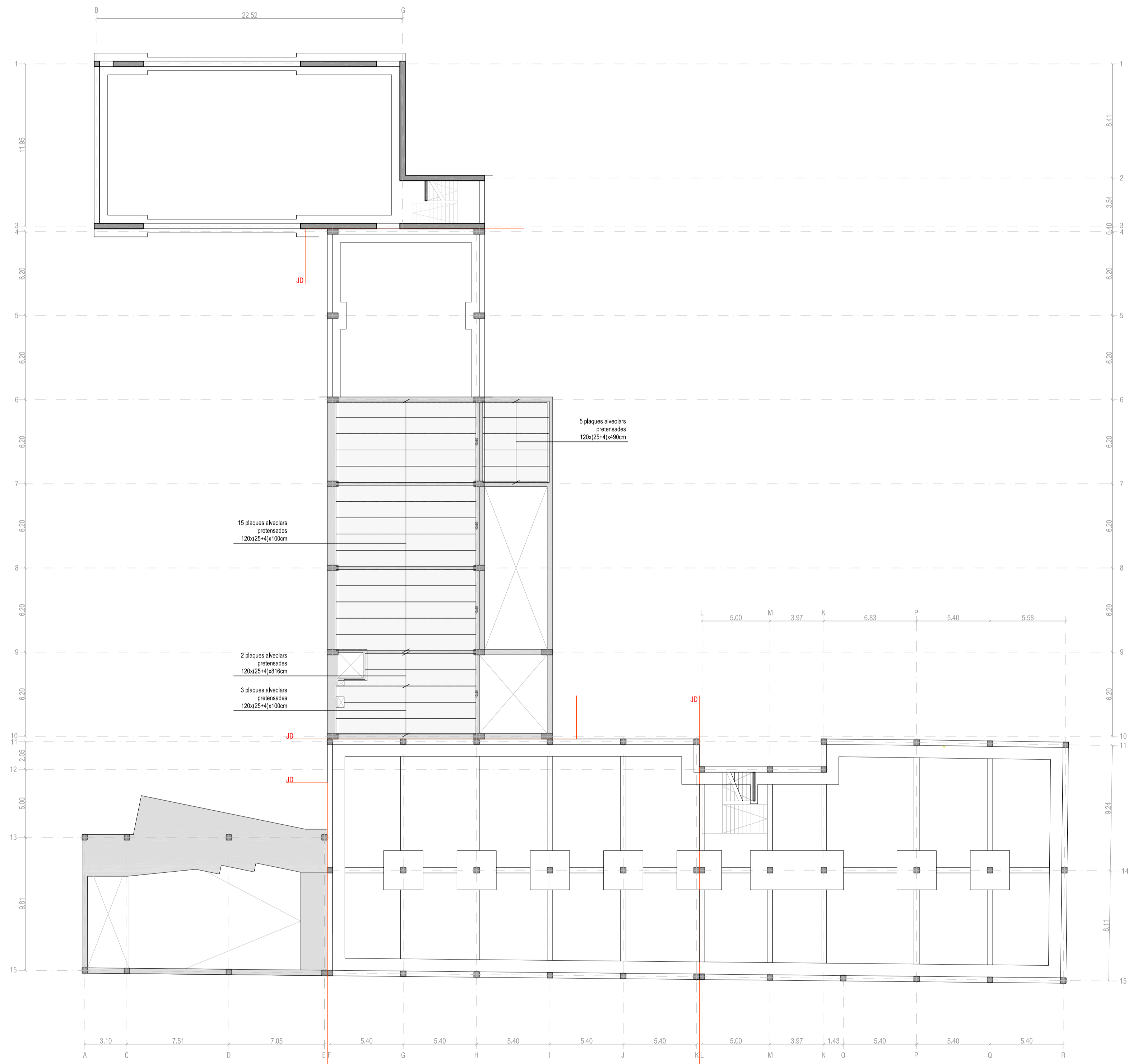
FONAMENTACIÓ-SOSTRE P-1
