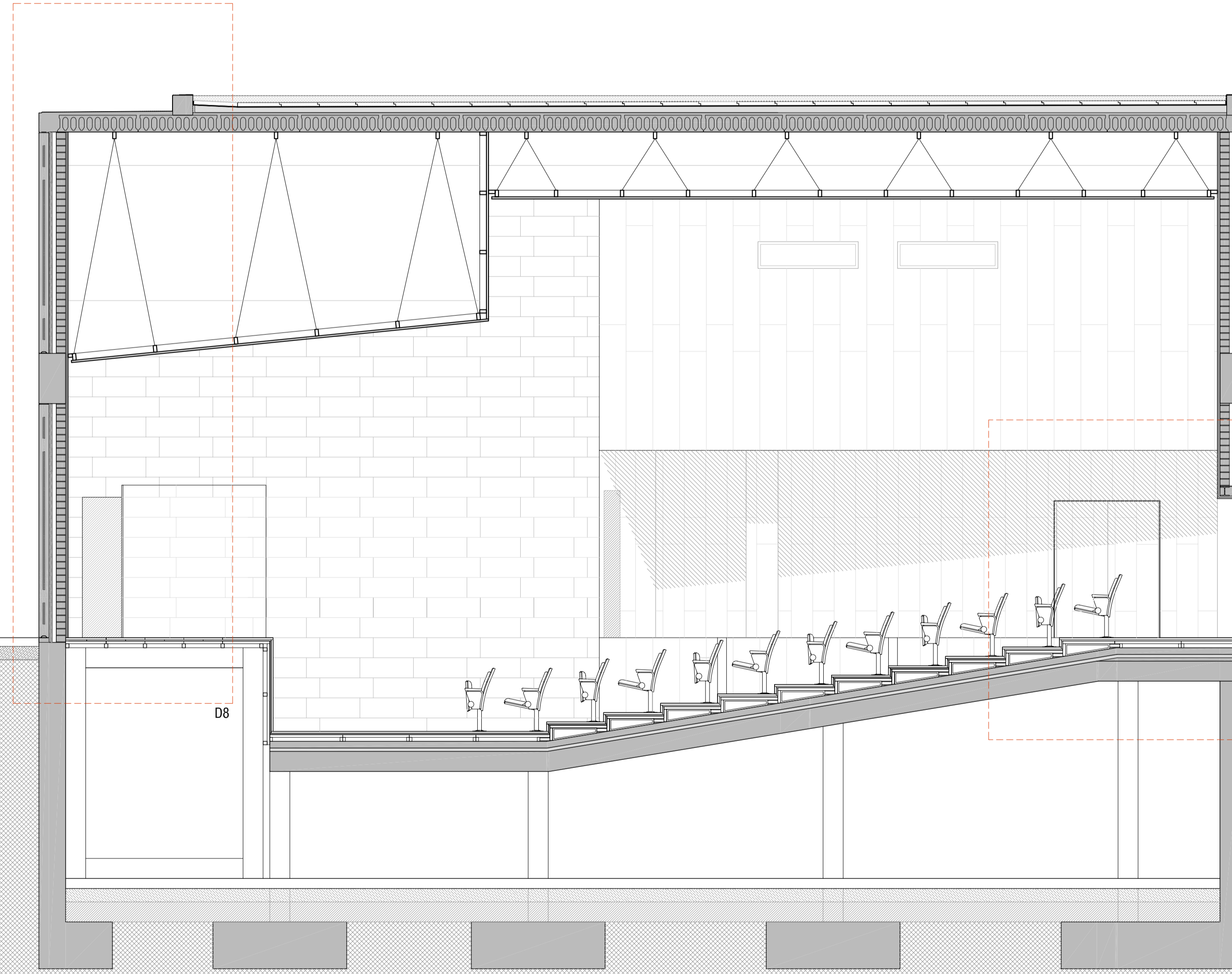
SECCIÓ A9 1/50
