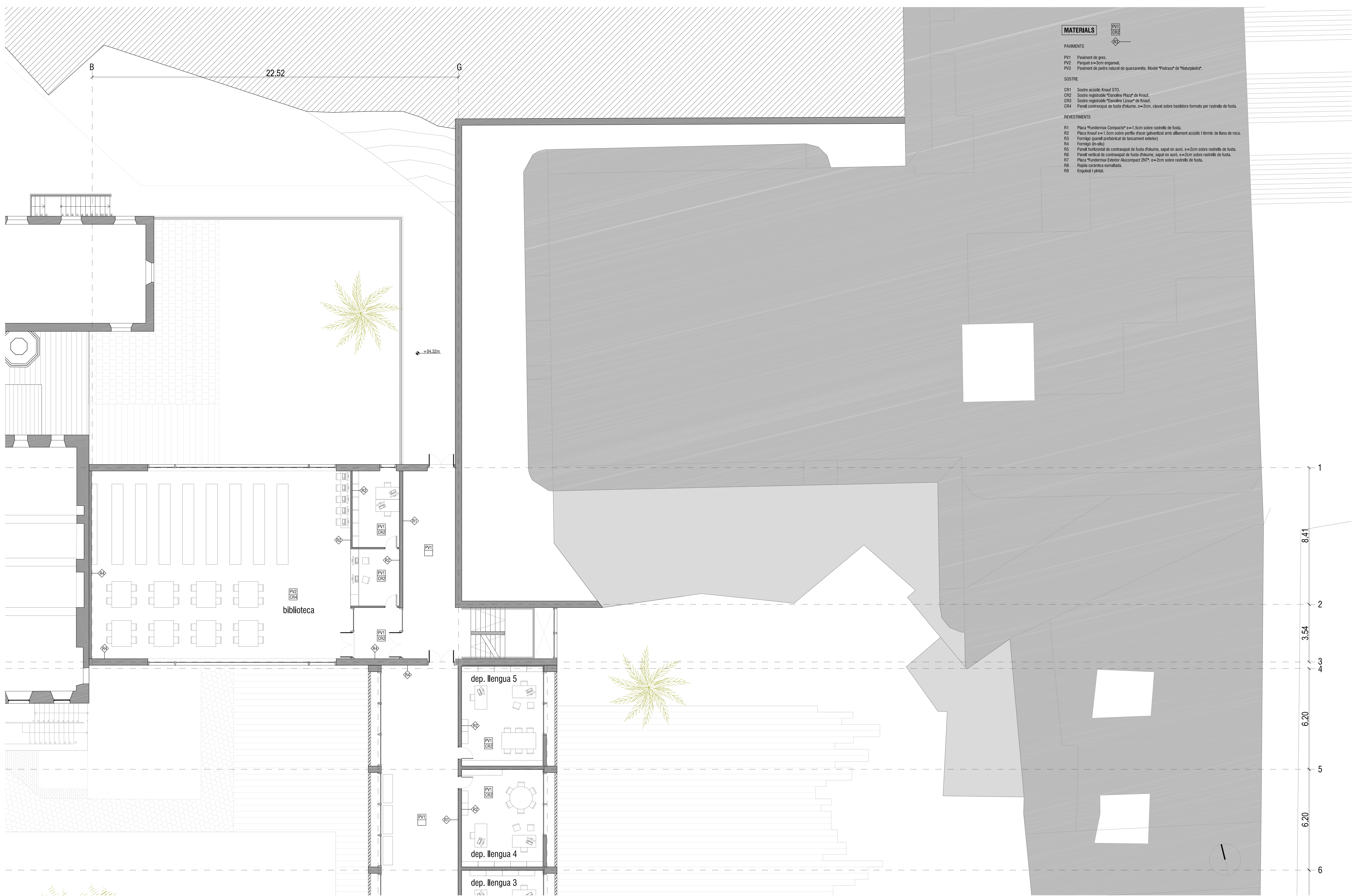
C04 - PLANTA PRIMERA, DETALL e. 1/100
