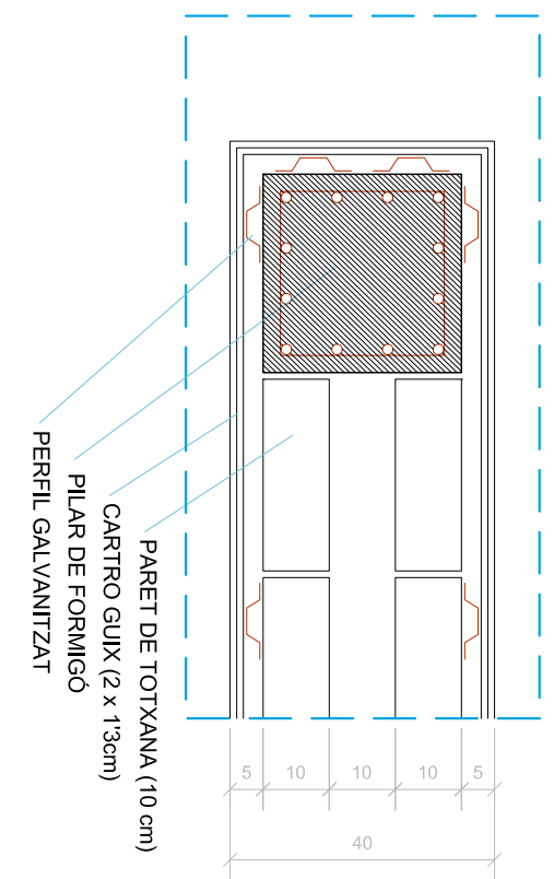
PARAMENTS INTERIORS E: 1/10
