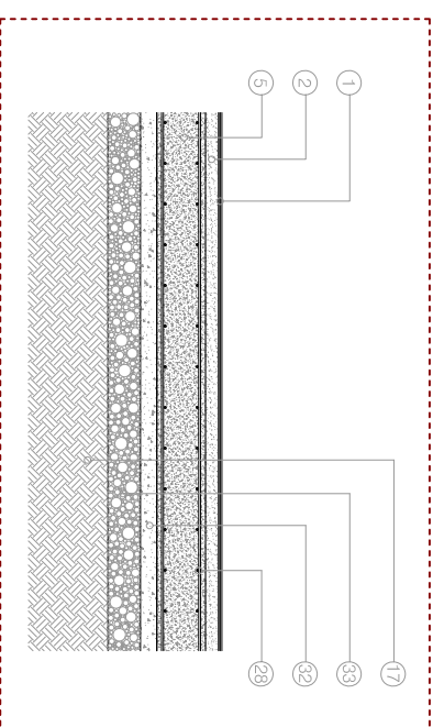
10. Detall paviment planta baixa.
