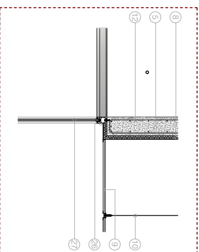
7. Detall tancament superior pati interior.
