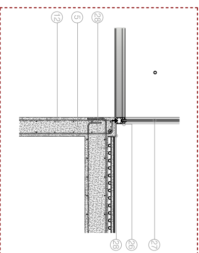
8. Detall tancament inferior pati interior.
