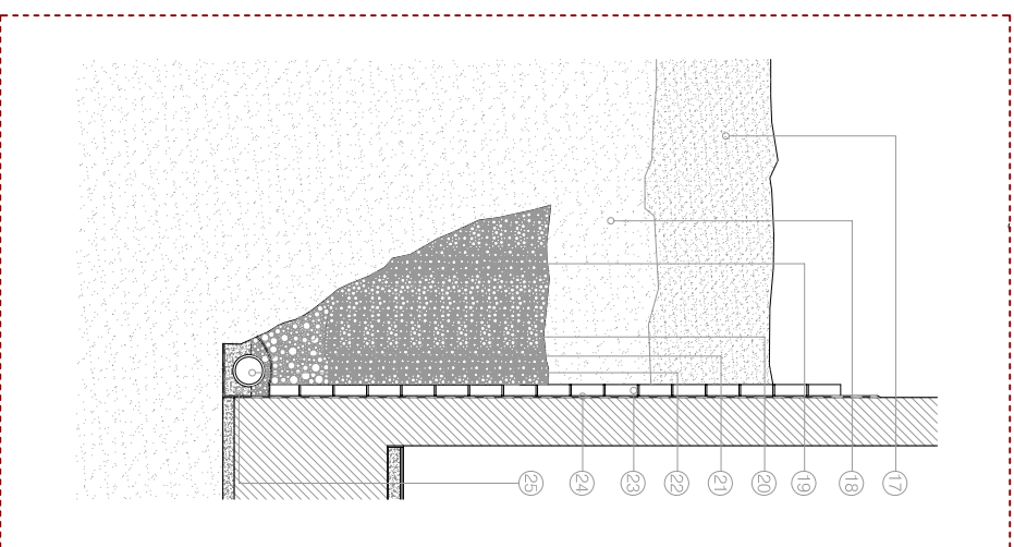
6. Detall drenatge mur de contacte.
