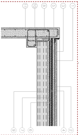
1. Detall coberta. Troçada amb façana lateral.
