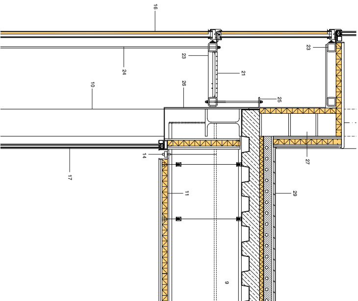
D1 SECCION VERTICAL_E 1/20
