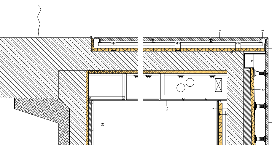
D05 SECCION VERTICAL DEL MURO PERIMETRAL, E:1/20
