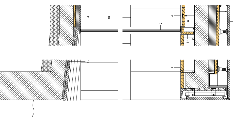
D06 SECCION VERTICAL ABERTURA EN EL MURO, E:1/20
