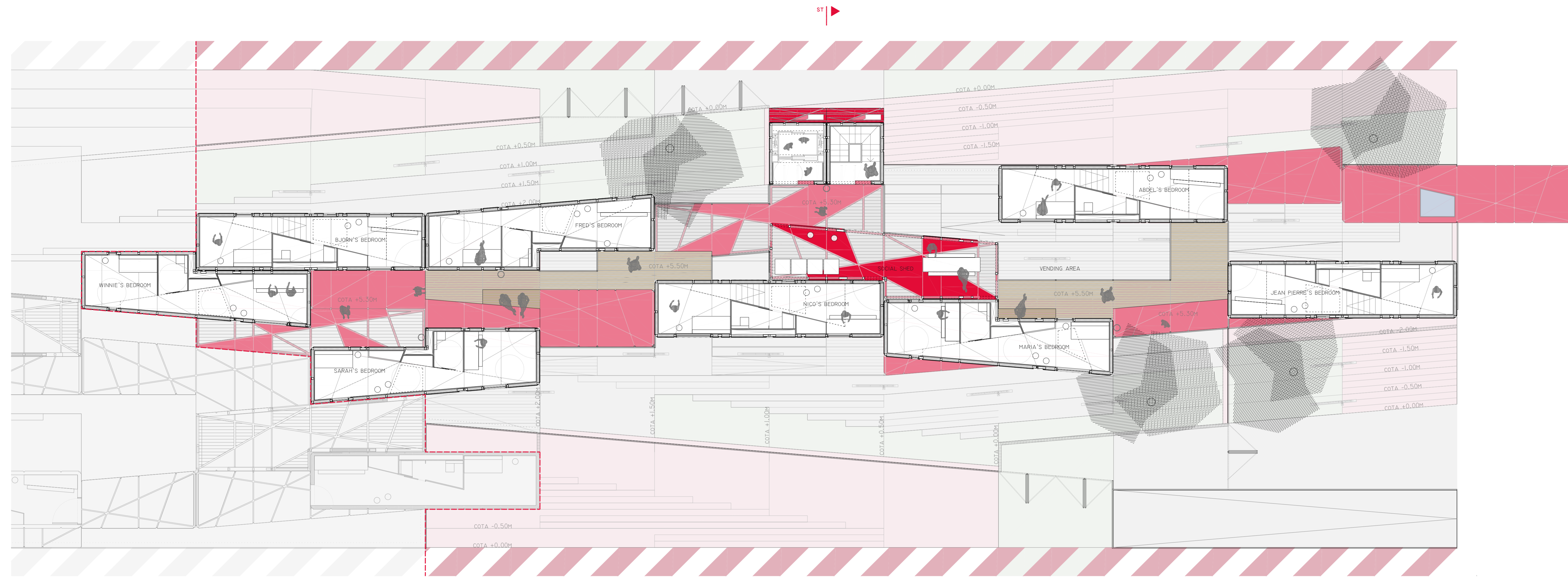
PLANTA CÀPSULES N2 E 1:100
