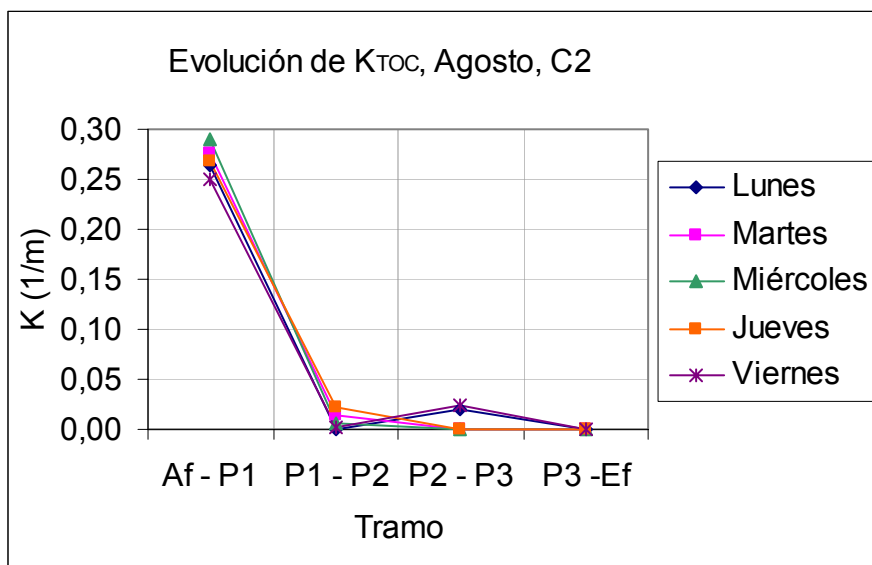
Figura A.2.2.3: Evolución de K_{TOC} en el humedal C2 según los datos obtenidos en el muestreo correspondiente a la campaña de agosto.
