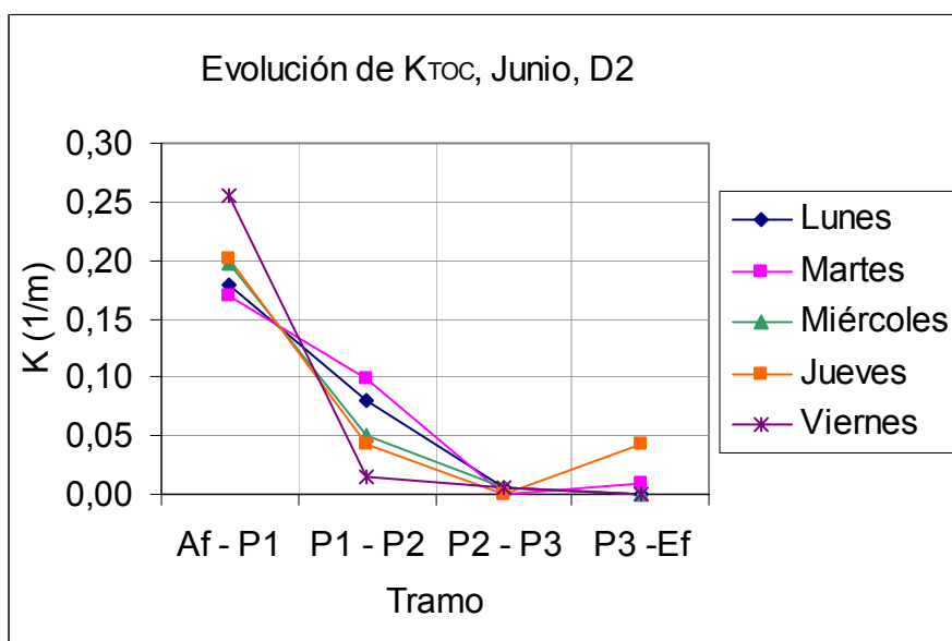
Figura A.2.2.5: Evolución de K_{TOC} en el humedal D2 según los datos obtenidos en el muestreo correspondiente a la campaña de junio.
