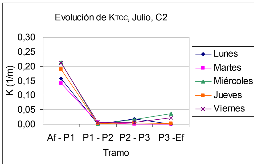
Figura A.2.2.2: Evolución de K_{TOC} en el humedal C2 según los datos obtenidos en el muestreo correspondiente a la campaña de julio.
