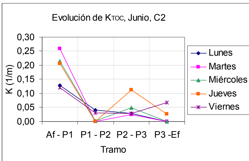
Figura A.2.2.1: Evolución de K_{TOC} en el humedal C2 según los datos obtenidos en el muestreo correspondiente a la campaña de junio.
