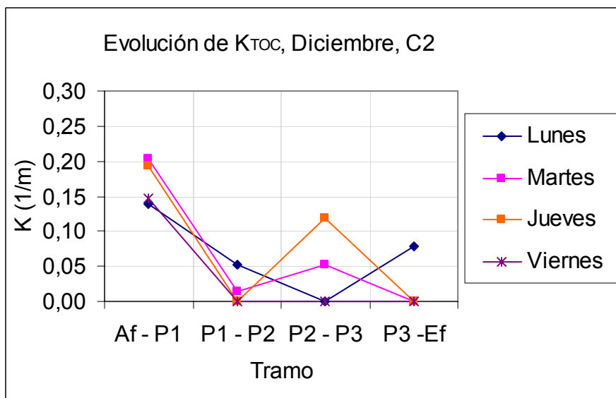
Figura A.2.2.4: Evolución de K_{TOC} en el humedal C2 según los datos obtenidos en el muestreo correspondiente a la campaña de diciembre.
