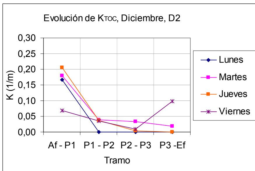
Figura A.2.2.6: Evolución de K_{TOC} en el humedal D2 según los datos obtenidos en el muestreo correspondiente a la campaña de diciembre.
