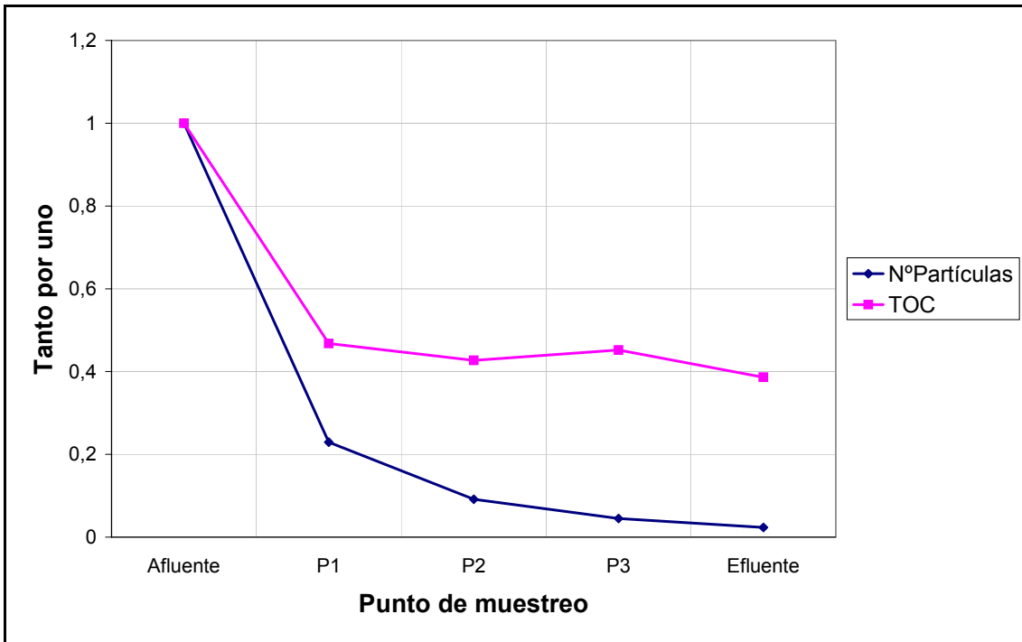
Figura A.2.1.11: Eliminación del número total de partículas y el TOC a lo largo del humedal C2, correspondiente al jueves de la campaña de junio.
