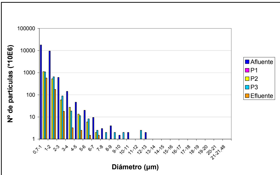
Figura A.2.1.27: Evolución del número de partículas según rangos de diámetros a lo largo del humedal D2, correspondiente al jueves de la campaña de junio.
