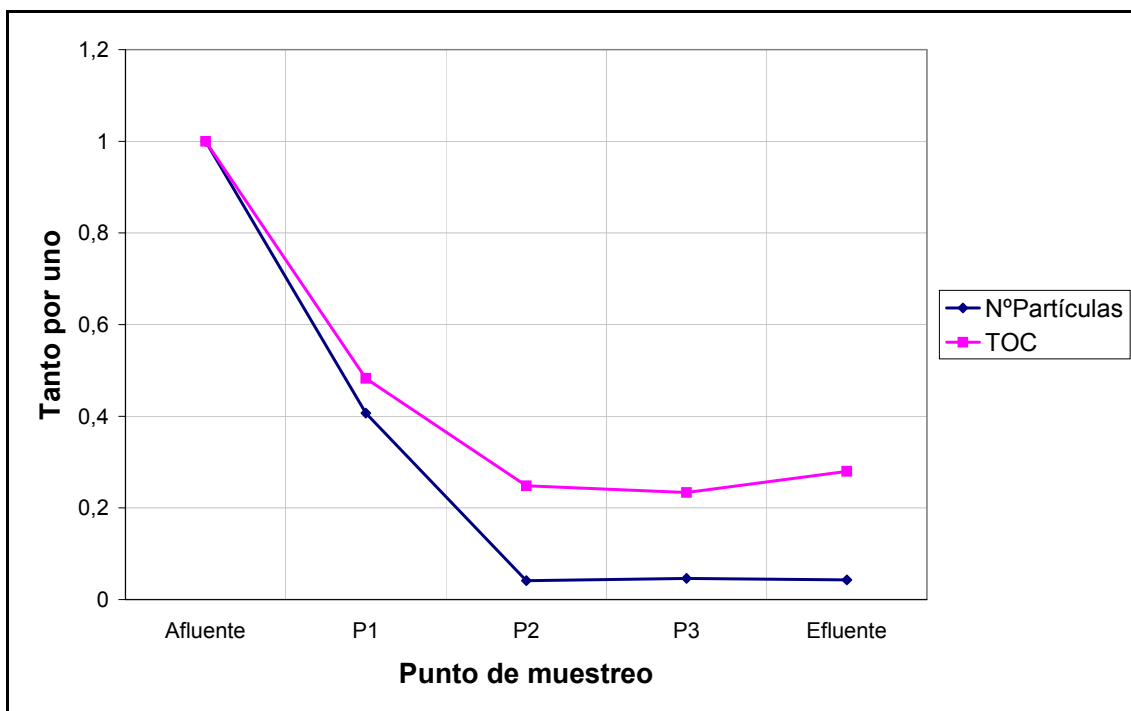
Figura A.2.1.17: Eliminación del número total de partículas y el TOC a lo largo del humedal D2, correspondiente al lunes de la campaña de junio.
