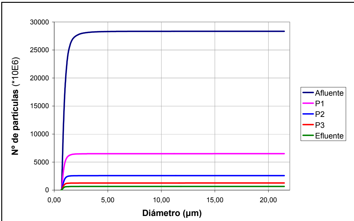
Figura A.2.1.10: Distribución acumulada de partículas en los distintos puntos de muestreo del humedal C2 correspondiente al jueves de la campaña de junio.
