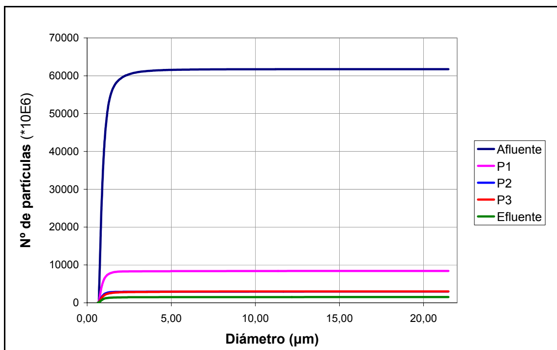
Figura A.2.1.1: Distribución acumulada de partículas en los distintos puntos de muestreo del humedal C2 correspondiente al lunes de la campaña de junio.
