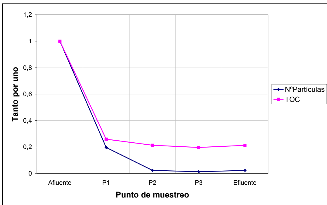
Figura A.2.1.29: Eliminación del número total de partículas y el TOC a lo largo del humedal D2, correspondiente al viernes de la campaña de junio.
