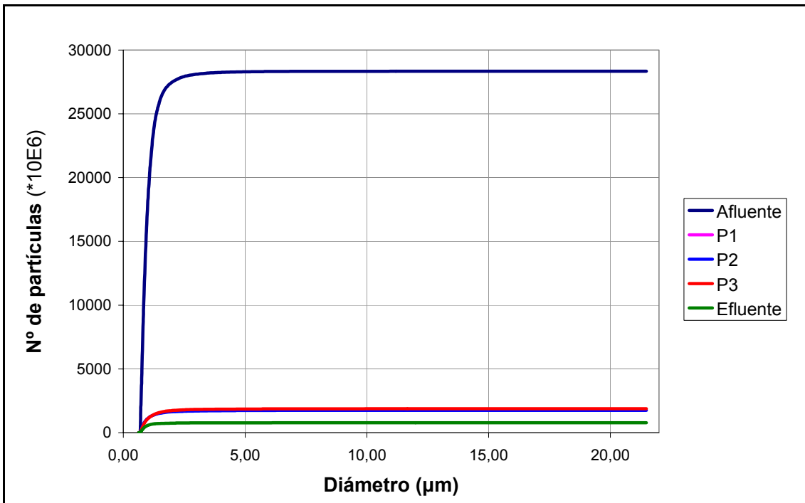
Figura A.2.1.25: Distribución acumulada de partículas en los distintos puntos de muestreo del humedal D2 correspondiente al jueves de la campaña de junio.
