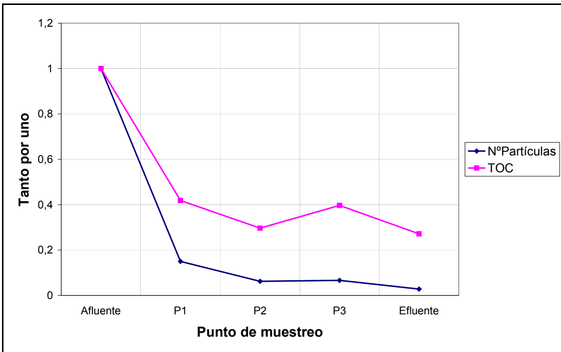
Figura A.2.1.26: Eliminación del número total de partículas y el TOC a lo largo del humedal D2, correspondiente al jueves de la campaña de junio.
