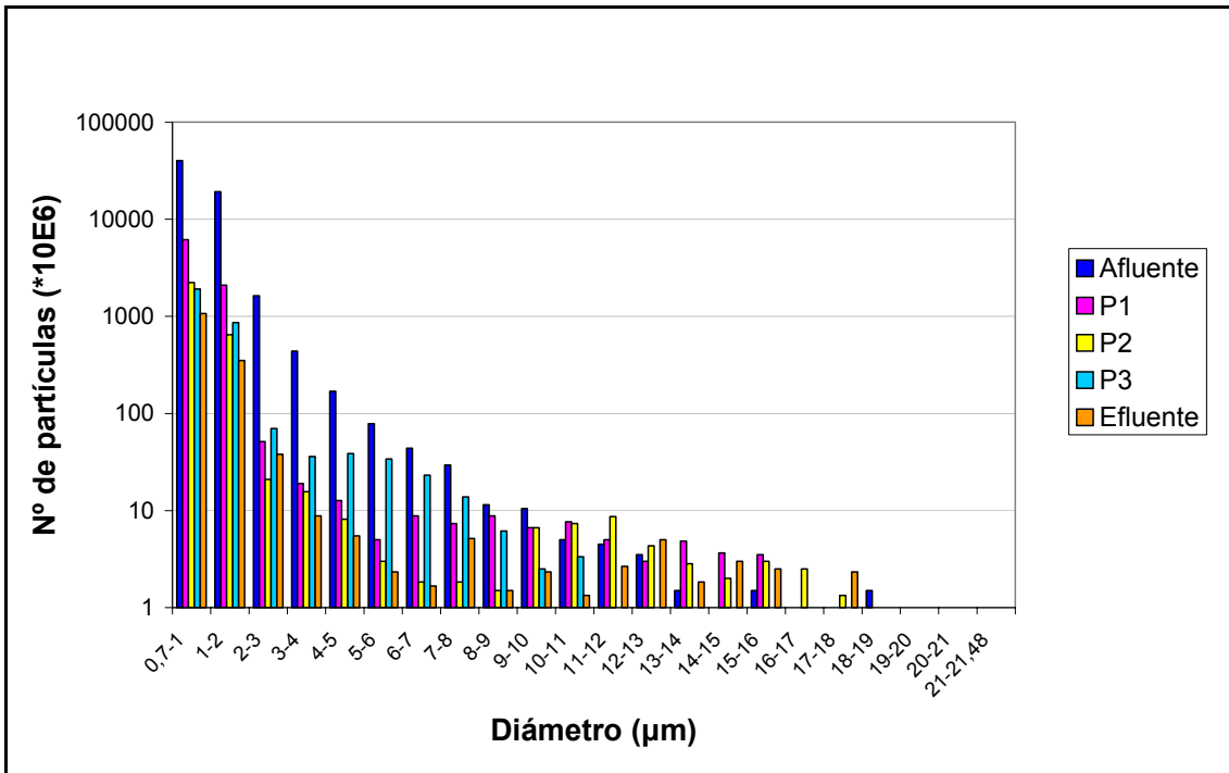
Figura A.2.1.3: Evolución del número de partículas según rangos de diámetros a lo largo del humedal C2, correspondiente al lunes de la campaña de junio.
