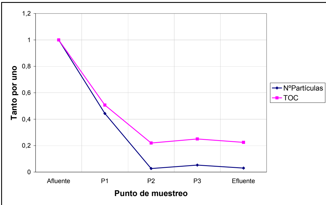
Figura A.2.1.20: Eliminación del número total de partículas y el TOC a lo largo del humedal D2, correspondiente al martes de la campaña de junio.
