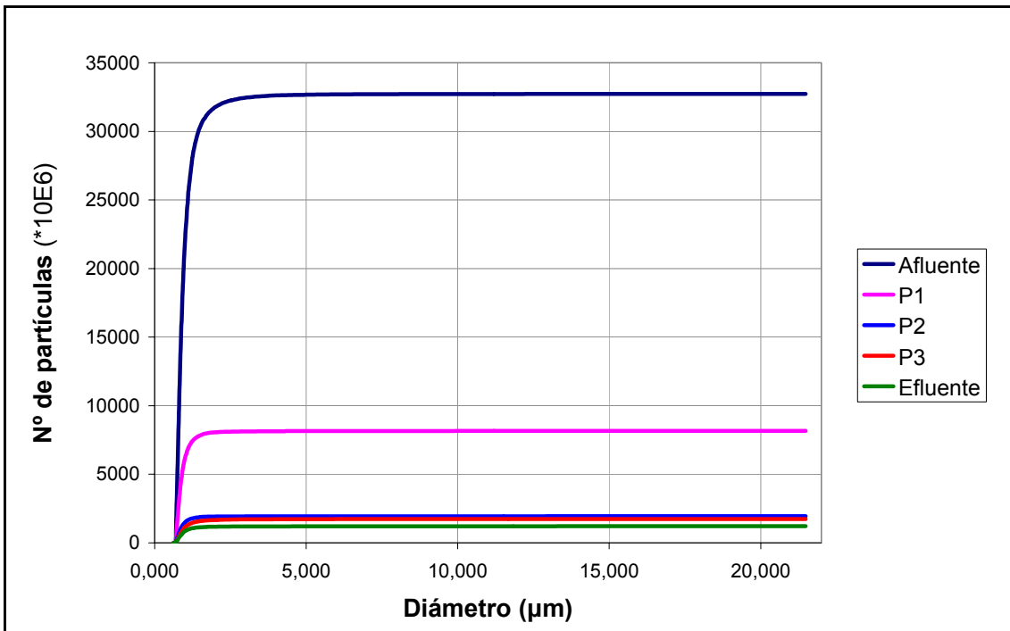
Figura A.2.1.4: Distribución acumulada de partículas en los distintos puntos de muestreo del humedal C2 correspondiente al martes de la campaña de junio.
