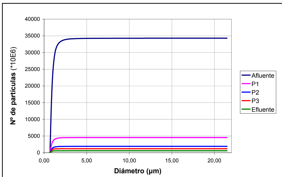
Figura A.2.1.13: Distribución acumulada de partículas en los distintos puntos de muestreo del humedal C2 correspondiente al viernes de la campaña de junio.
