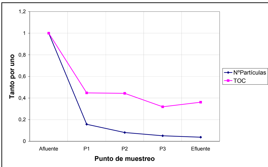
Figura A.2.1.8: Eliminación del número total de partículas y el TOC a lo largo del humedal C2, correspondiente al miércoles de la campaña de junio.
