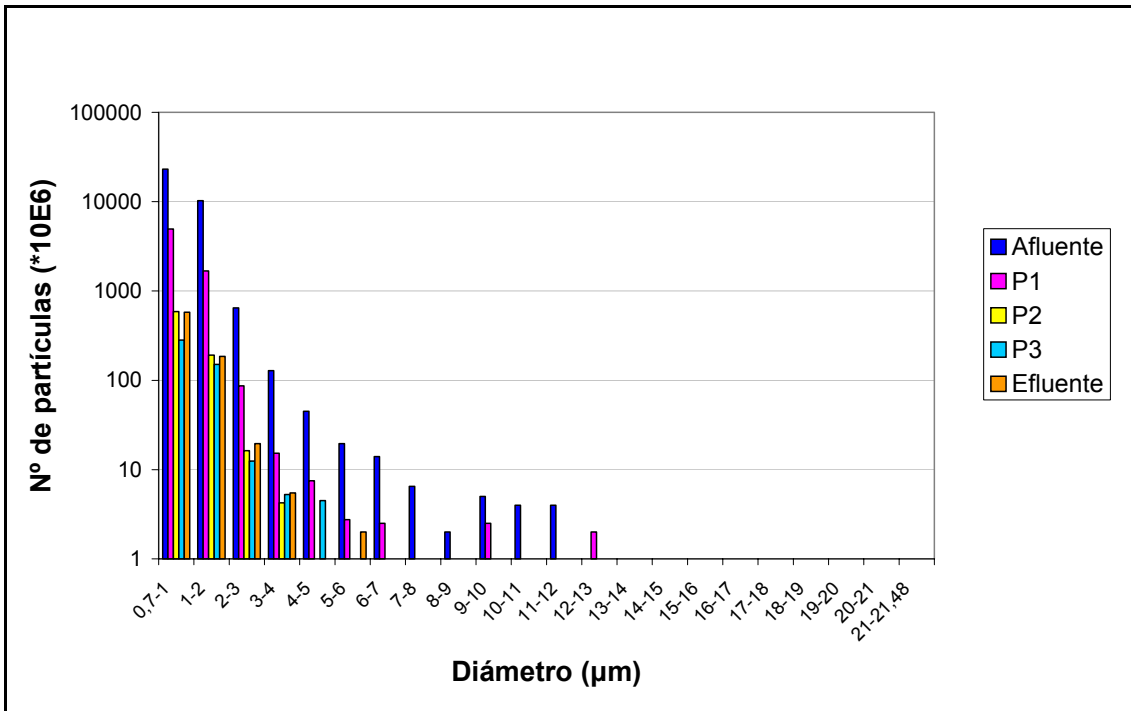
Figura A.2.1.30: Evolución del número de partículas según rangos de diámetros a lo largo del humedal D2, correspondiente al viernes de la campaña de junio.
