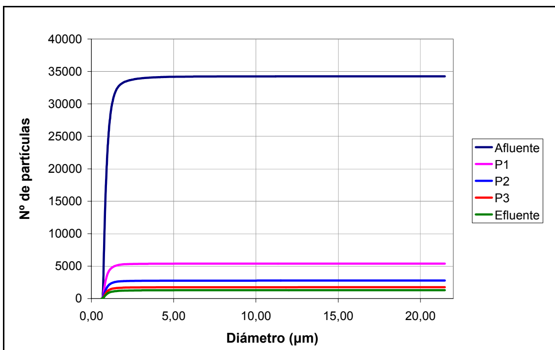
Figura A.2.1.7: Distribución acumulada de partículas en los distintos puntos de muestreo del humedal C2 correspondiente al miércoles de la campaña de junio.
