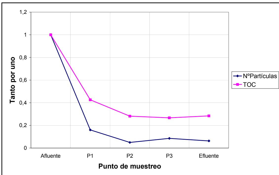
Figura A.2.1.23: Eliminación del número total de partículas y el TOC a lo largo del humedal D2, correspondiente al miércoles de la campaña de junio.
