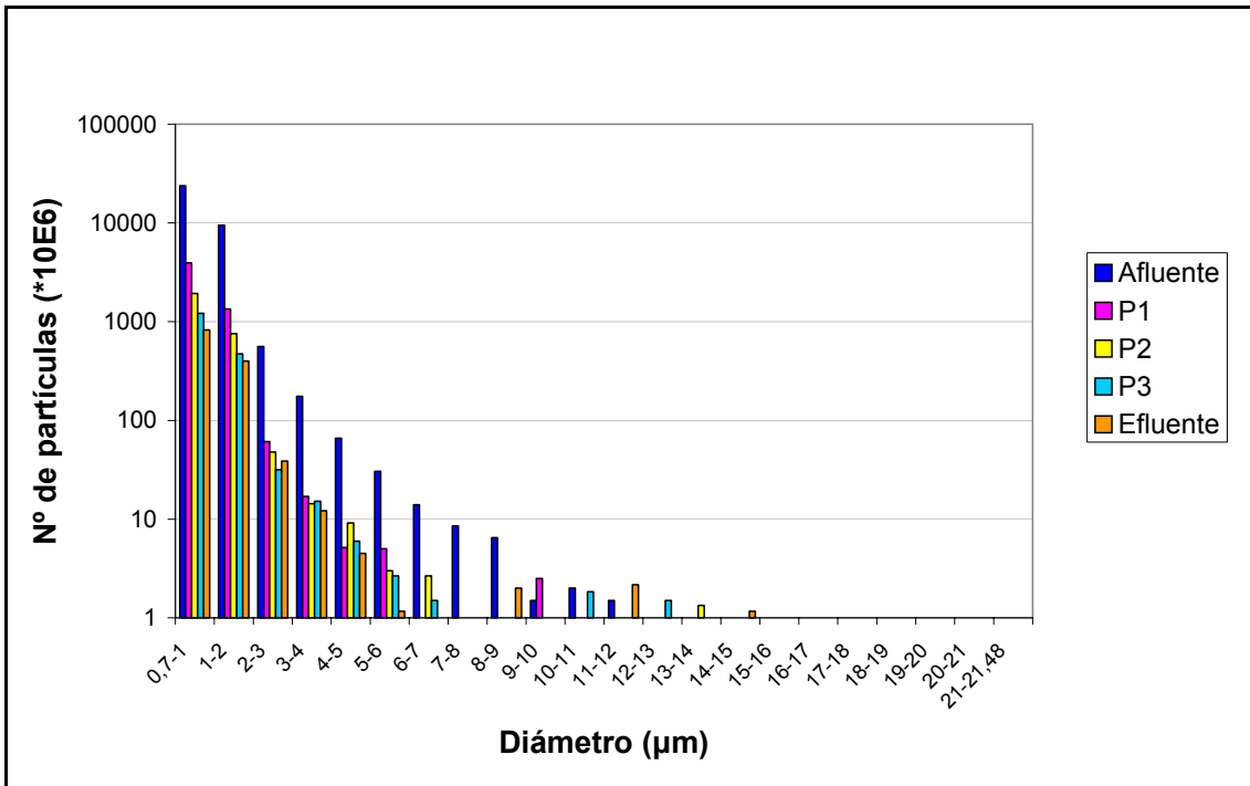
Figura A.2.1.9: Evolución del número de partículas según rangos de diámetros a lo largo del humedal C2, correspondiente al miércoles de la campaña de junio.
