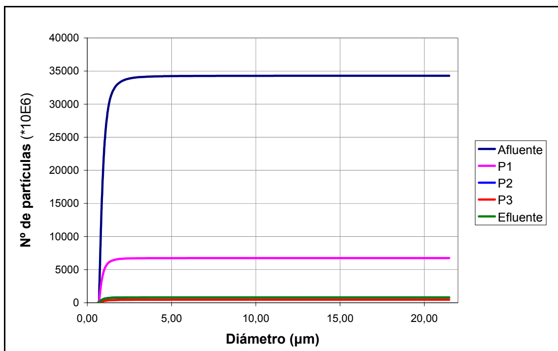
Figura A.2.1.28: Distribución acumulada de partículas en los distintos puntos de muestreo del humedal D2 correspondiente al viernes de la campaña de junio.
