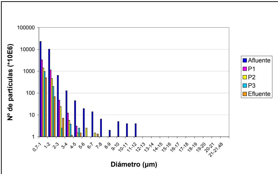
Figura A.2.1.15: Evolución del número de partículas según rangos de diámetros a lo largo del humedal C2, correspondiente al viernes de la campaña de junio.
