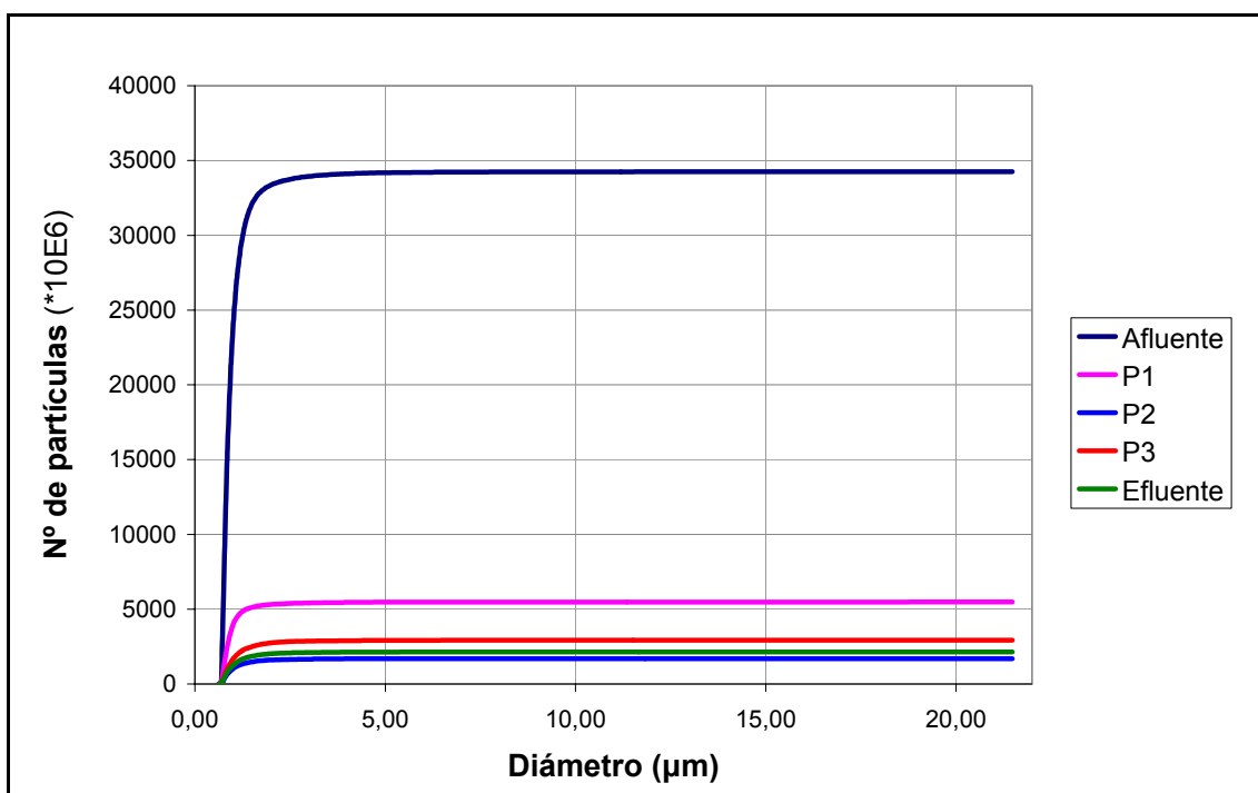
Figura A.2.1.22: Distribución acumulada de partículas en los distintos puntos de muestreo del humedal D2 correspondiente al miércoles de la campaña de junio.
