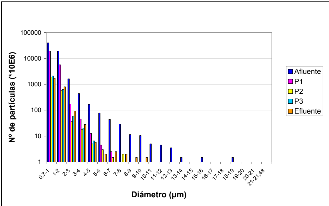
Figura A.2.1.18: Evolución del número de partículas según rangos de diámetros a lo largo del humedal D2, correspondiente al lunes de la campaña de junio.
