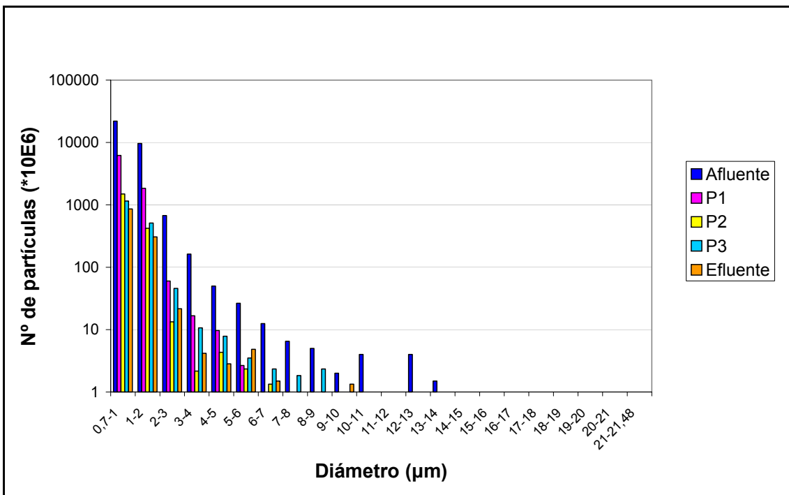
Figura A.2.1.6: Evolución del número de partículas según rangos de diámetros a lo largo del humedal C2, correspondiente al martes de la campaña de junio.
