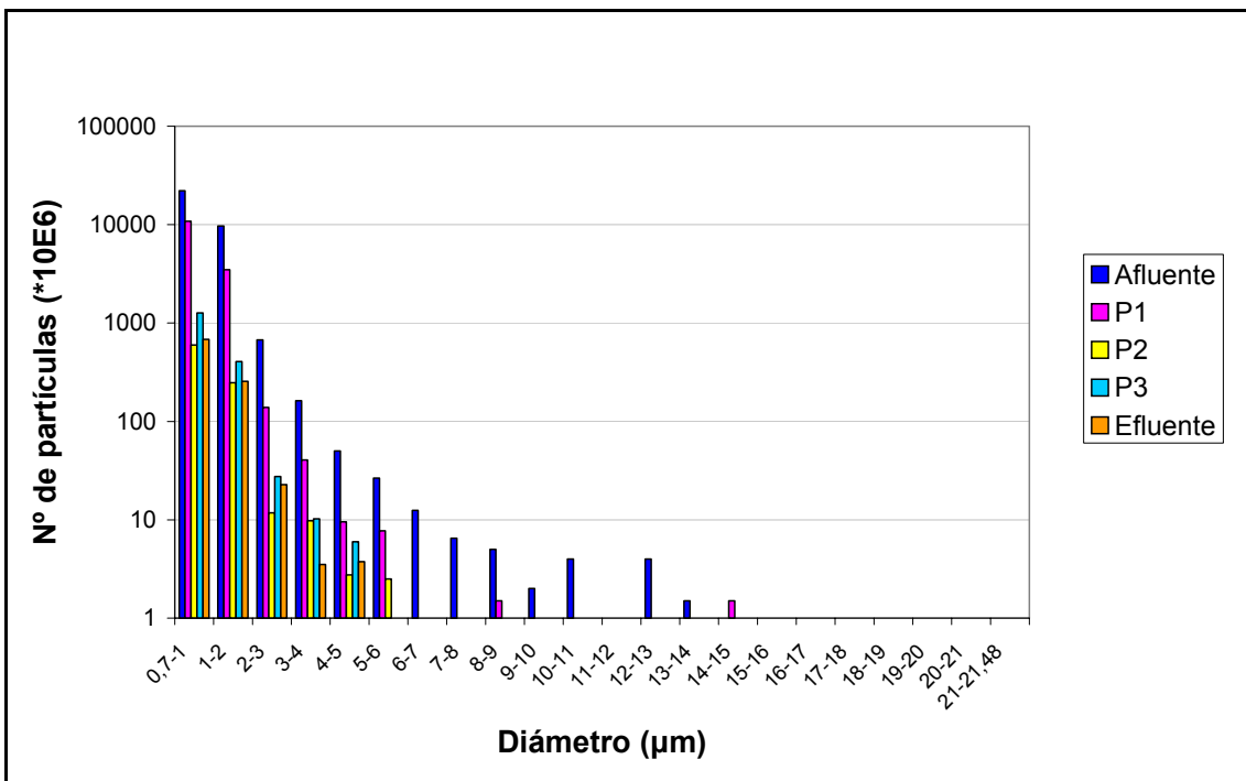
Figura A.2.1.21: Evolución del número de partículas según rangos de diámetros a lo largo del humedal D2, correspondiente al martes de la campaña de junio.
