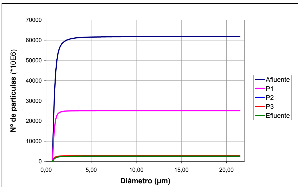
Figura A.2.1.16: Distribución acumulada de partículas en los distintos puntos de muestreo del humedal D2 correspondiente al lunes de la campaña de junio.
