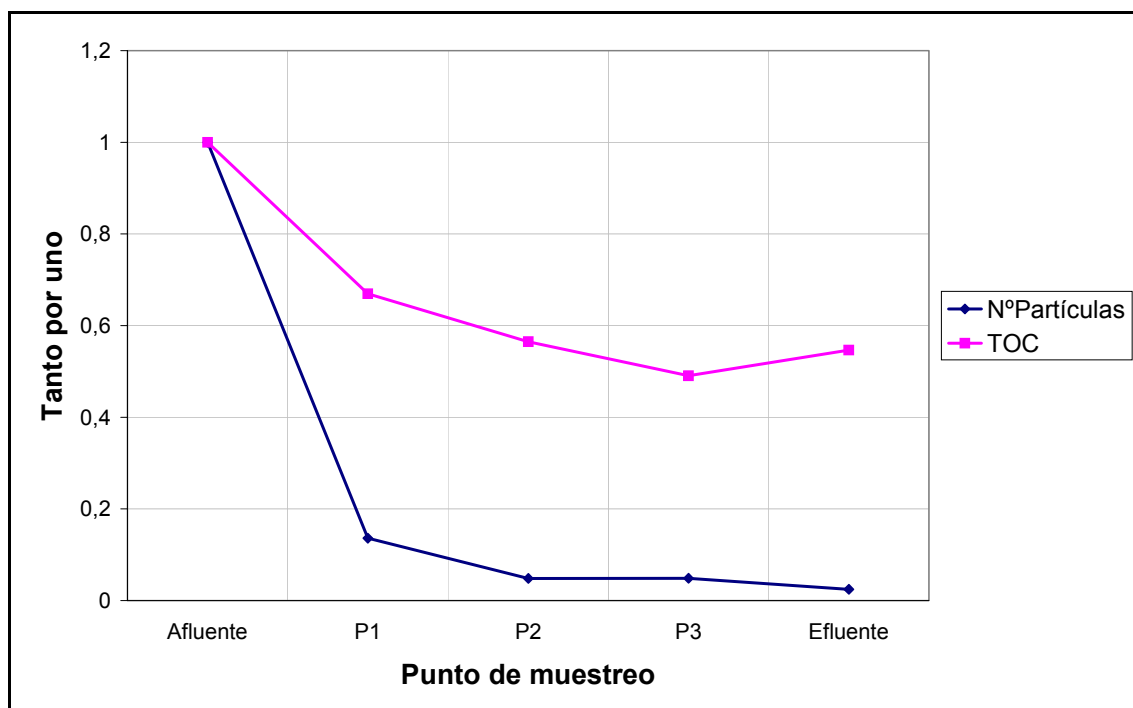
Figura A.2.1.2: Eliminación del número total de partículas y el TOC a lo largo del humedal C2, correspondiente al lunes de la campaña de junio.
