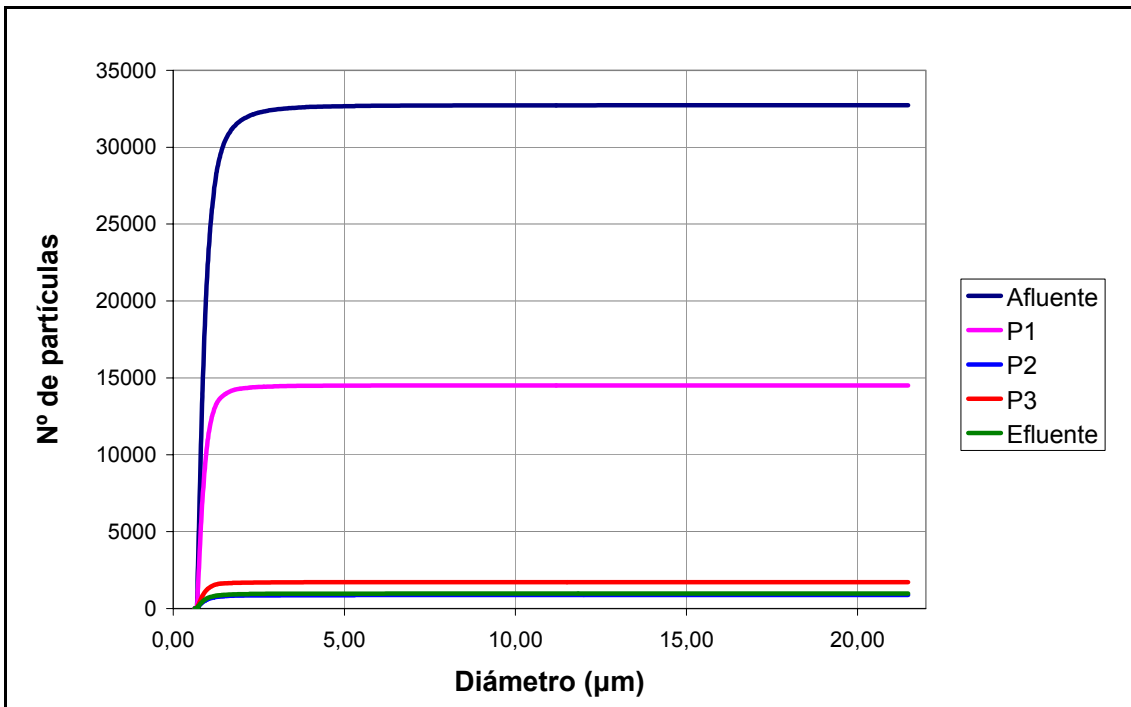
Figura A.2.1.19: Distribución acumulada de partículas en los distintos puntos de muestreo del humedal D2 correspondiente al martes de la campaña de junio.
