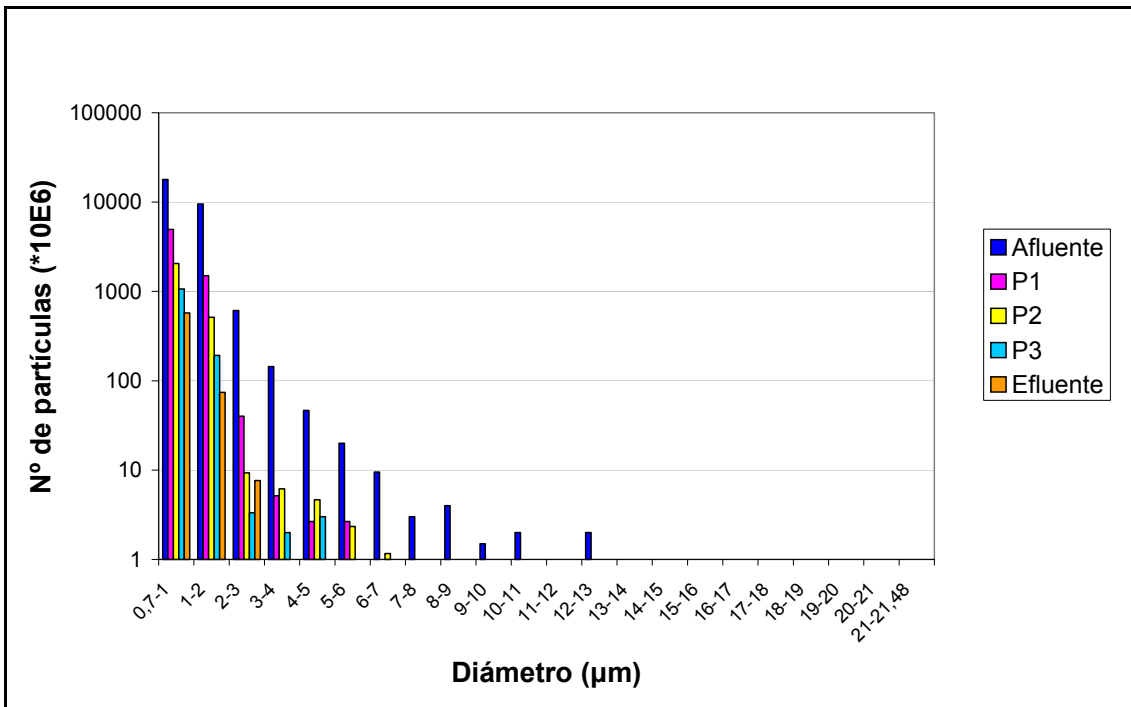
Figura A.2.1.12: Evolución del número de partículas según rangos de diámetros a lo largo del humedal C2, correspondiente al jueves de la campaña de junio.
