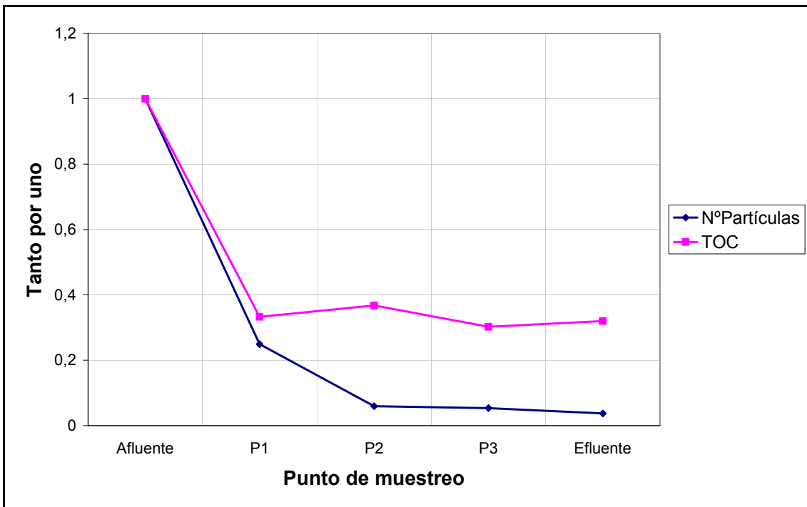
Figura A.2.1.5: Eliminación del número total de partículas y el TOC a lo largo del humedal C2, correspondiente al martes de la campaña de junio.
