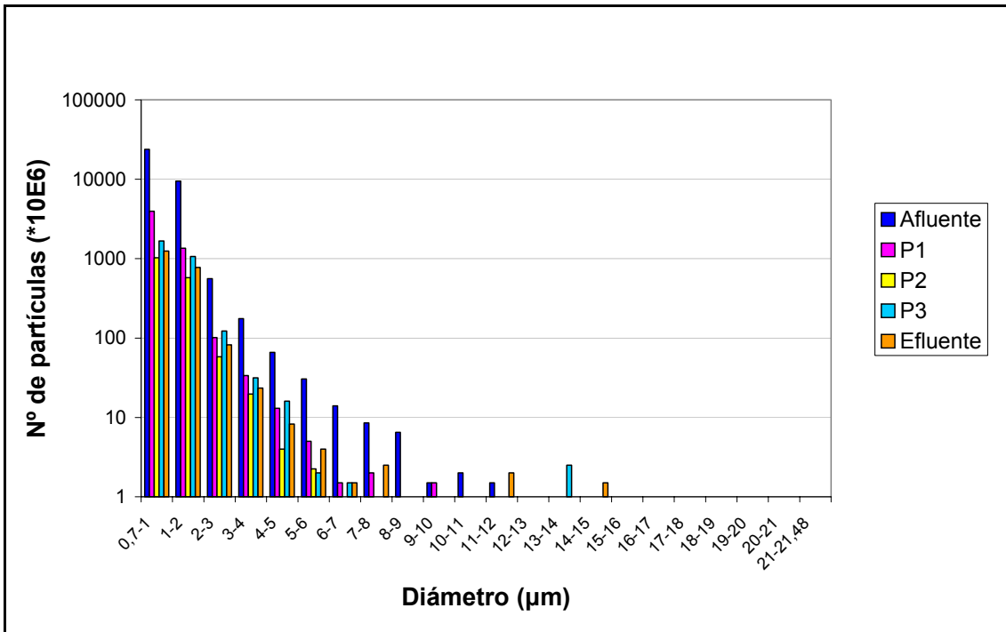
Figura A.2.1.24: Evolución del número de partículas según rangos de diámetros a lo largo del humedal D2, correspondiente al miércoles de la campaña de junio.
