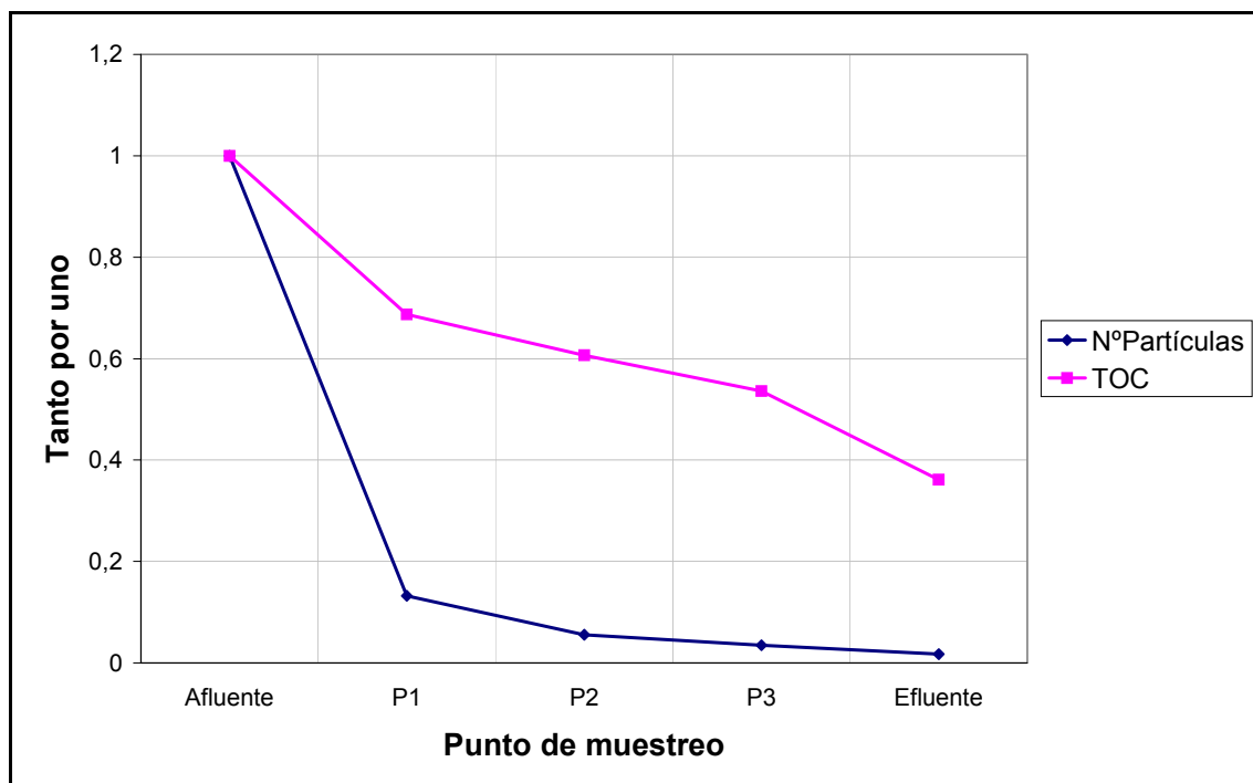
Figura A.2.1.14: Eliminación del número total de partículas y el TOC a lo largo del humedal C2, correspondiente al viernes de la campaña de junio.
