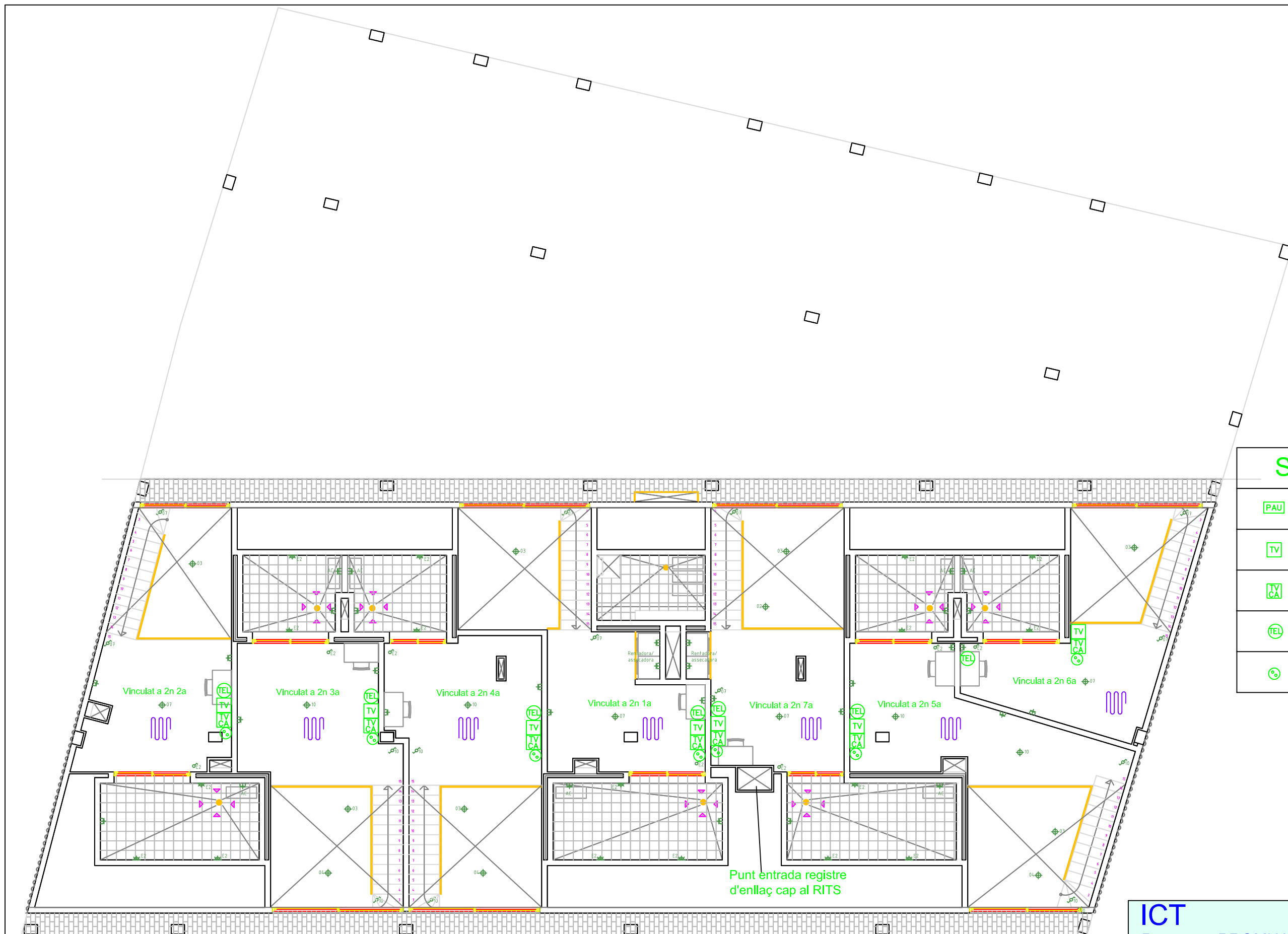
Planta Sotacoberta E=1:100
