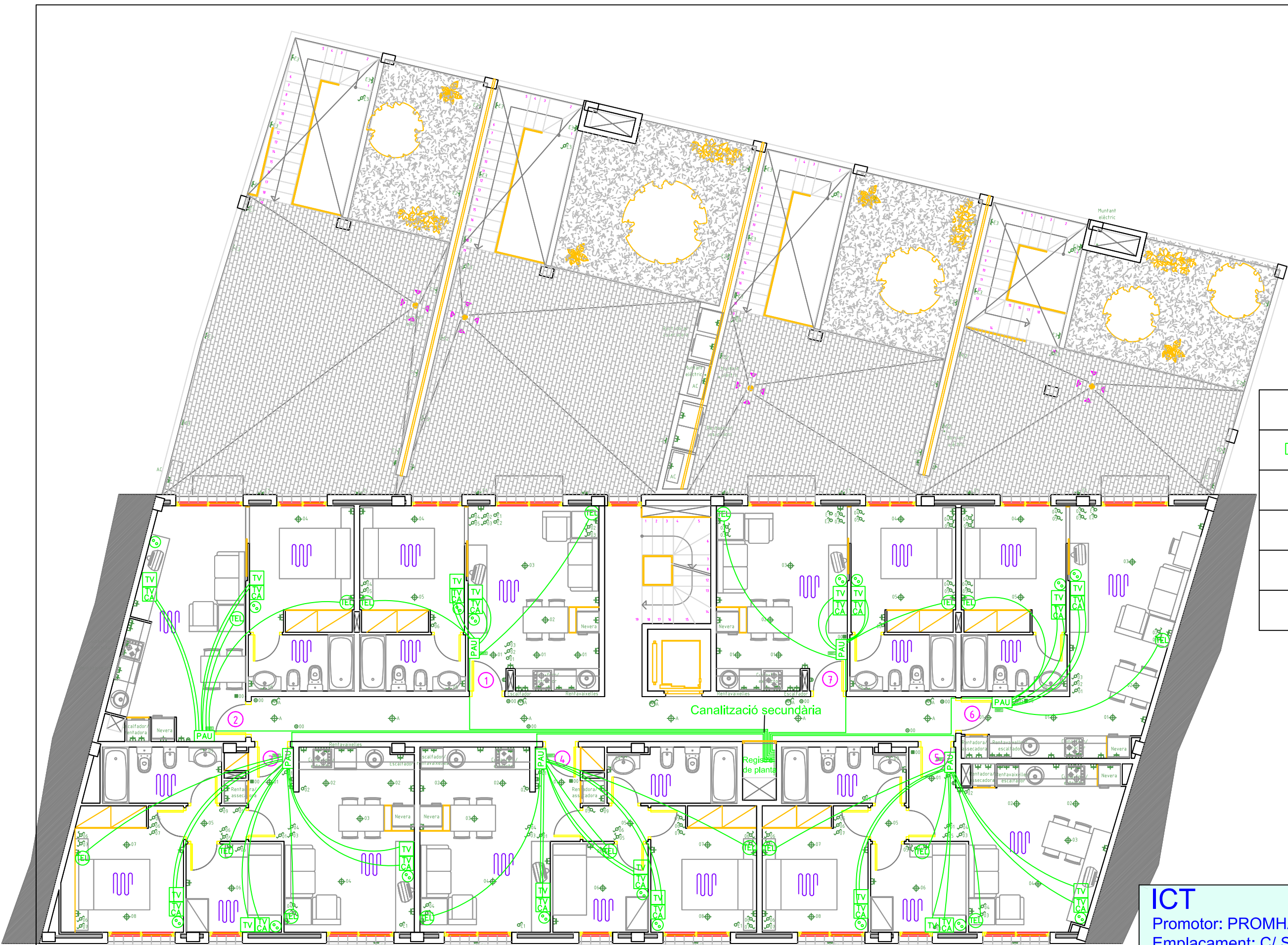
Planta Pisos 1a E=1:100
