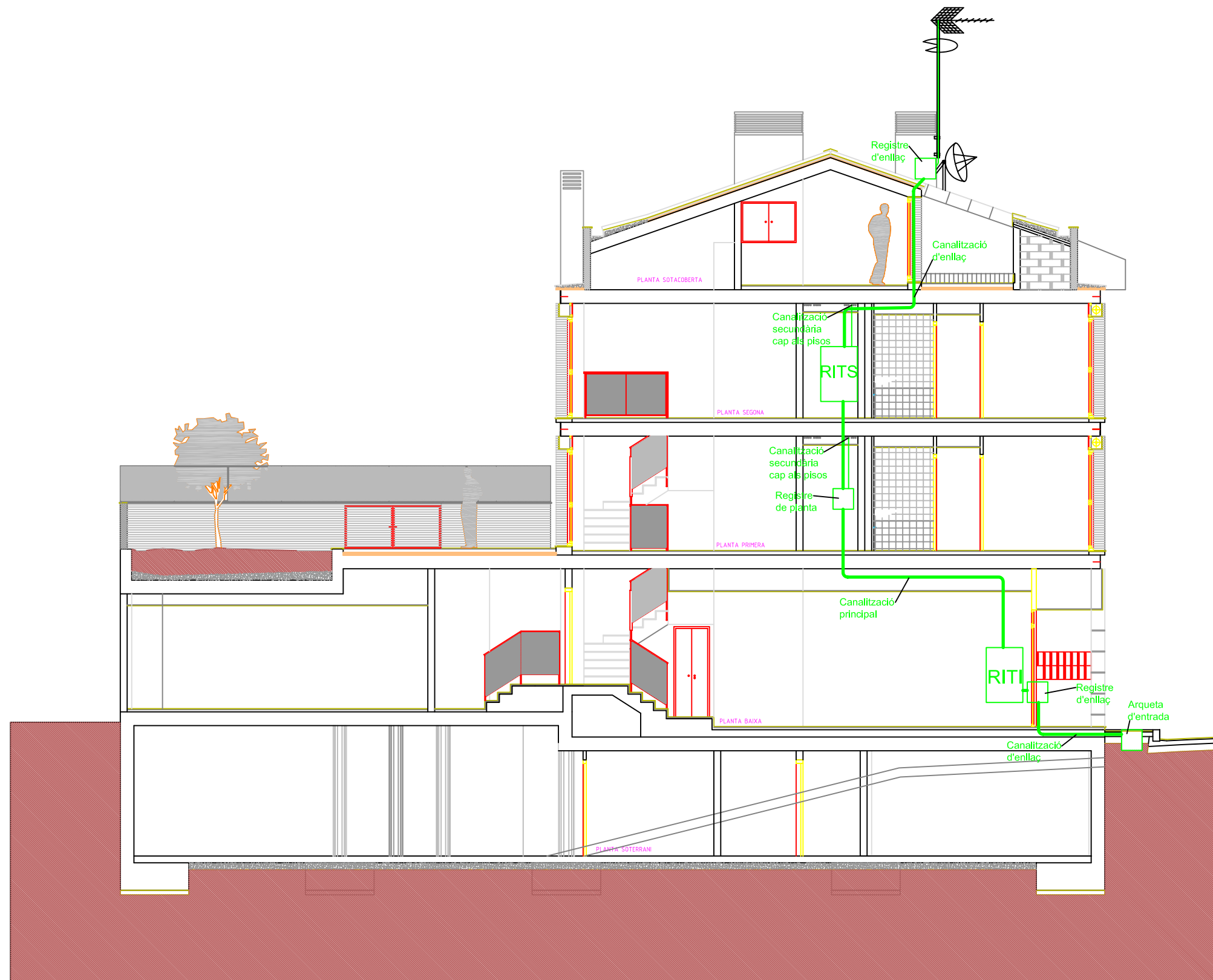
Secció, E = 1:200
